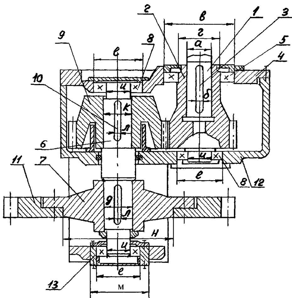
1 – переходник; 2 – шестерня; 3 – шпонка; 4 – крышка редуктора; 5 – подшипник; 6 – вал; 7 – ступица; 8 – подшипник; 9 – колесо; 10 – шпонка; 11 – венец; 12 – корпус редуктора; 13 – вкладыш
