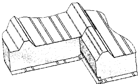
Стыковое соединение панелей ПКТМ
