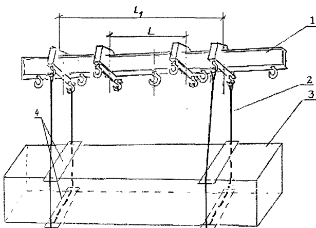
Схема строповки пакета при разгрузке автомобиля с использованием траверсы
