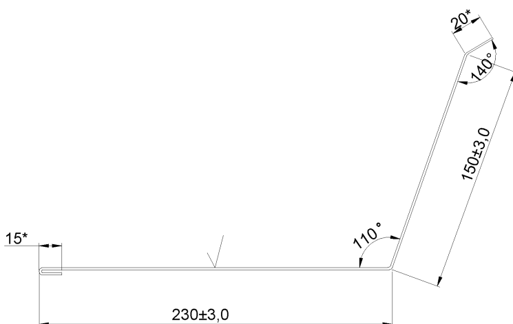
Рисунок Б.8 – Карниз (К)
