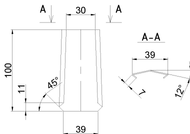
Рисунок Б.35 Замок 150 (З150)
