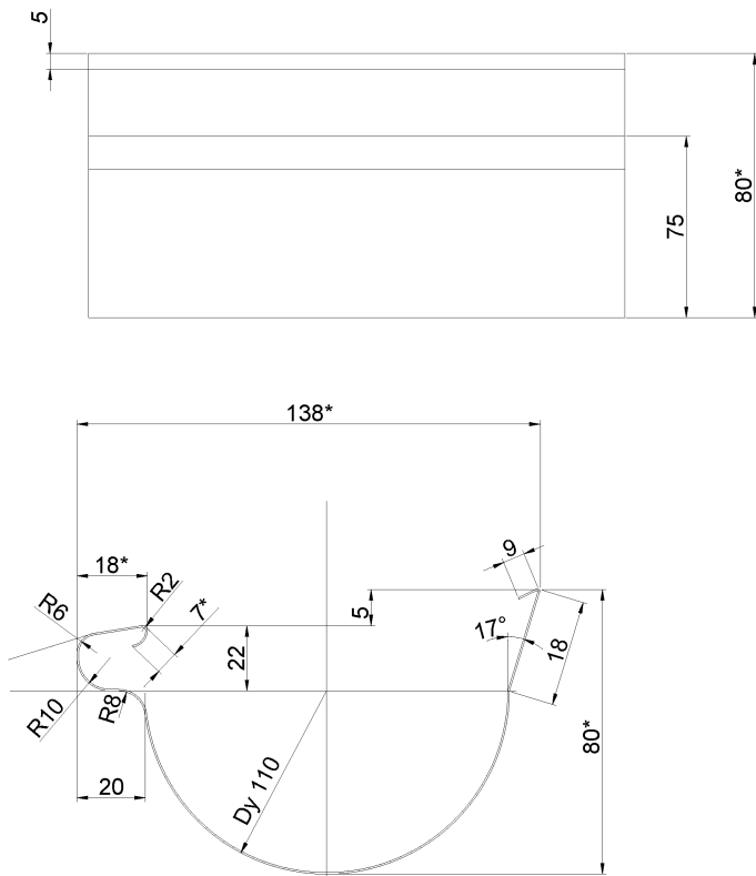
Рисунок Б.11 – Желоб 100 (Ж100)
