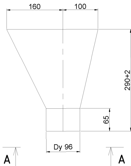
Рисунок Б.20 – Воронка (В100)
