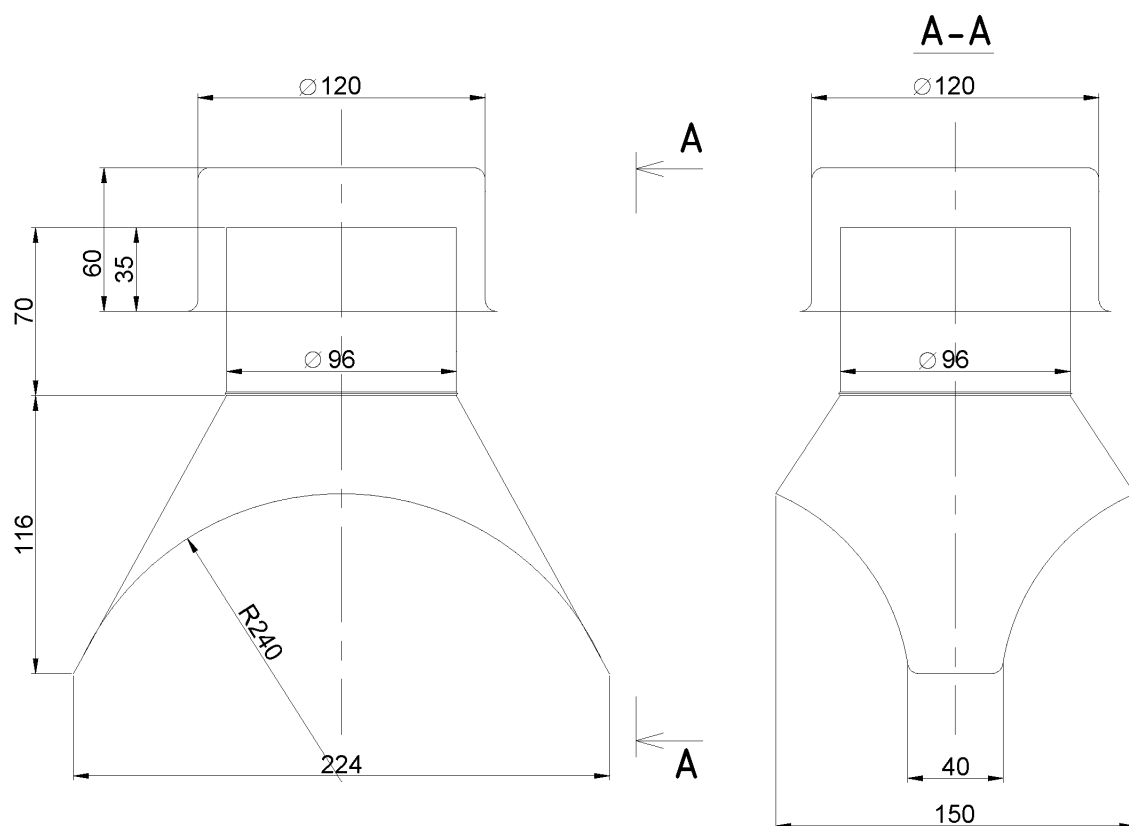
Рисунок Б.5 – Вентиляция конька (Вк)
