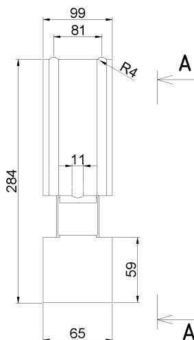
Рисунок Б.31 - Элемент желоба соединительный 150 (ЗЖС150)
