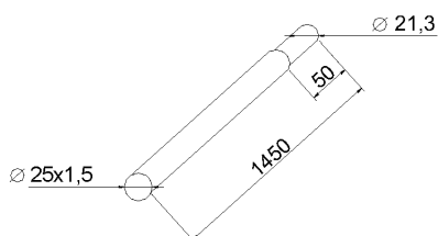
Рисунок Б.27 Труба снегозадержателя 1 (ТрСз/1)
