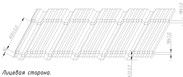
Рисунок 4 – металлочерепица «Shake» МЧ 43
