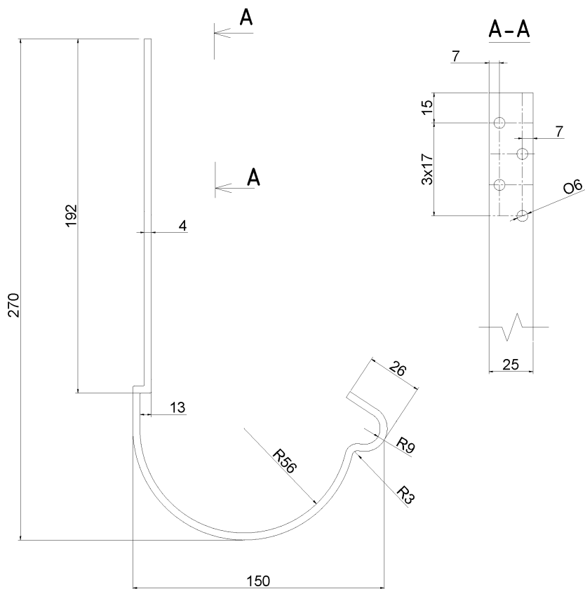
Рисунок Б.13 Держатель желоба 100 (Дж100)
