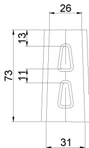
Рисунок Б.24 – Замок (З 100)
