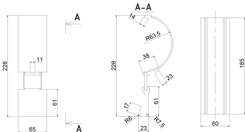
Рисунок Б.16 – Элемент желоба соединительный (ЗЖС100)
