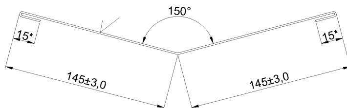
Рисунок Б.7 – Верхняя ендова (EB)
