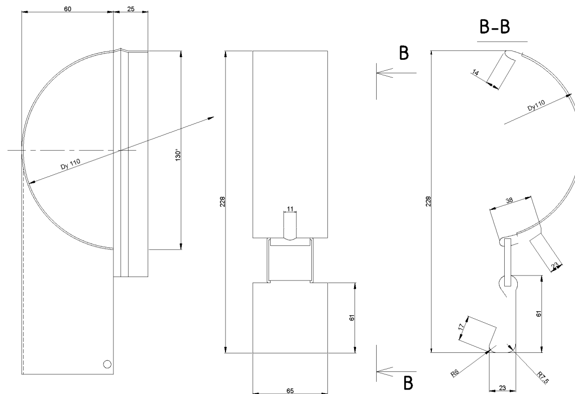
Рисунок Б.41 Комплект углового универсального желоба 100 (УЖ100)
