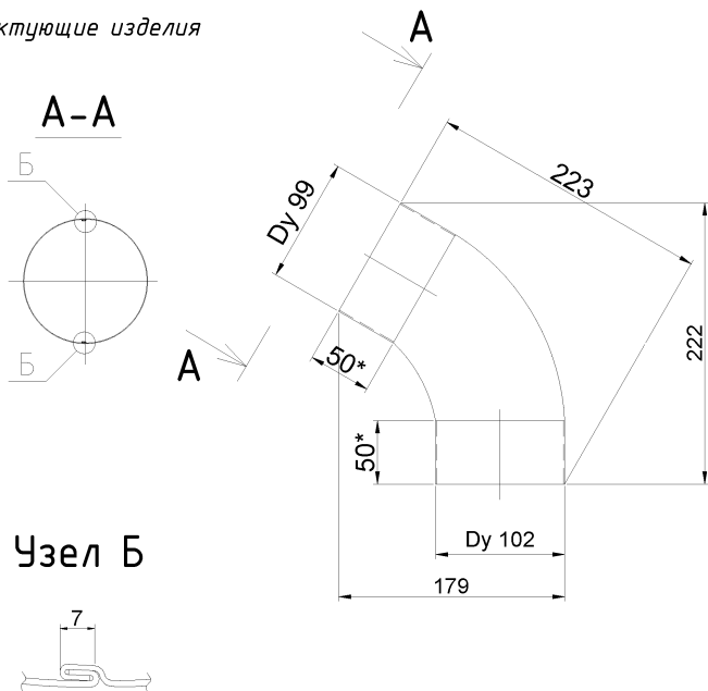
Рисунок Б.36 Колено угловое 100 (КУз100)
