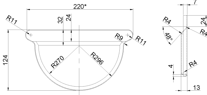
Рисунок Б.30 Заглушка желоба 150 (ЗЖ150)
