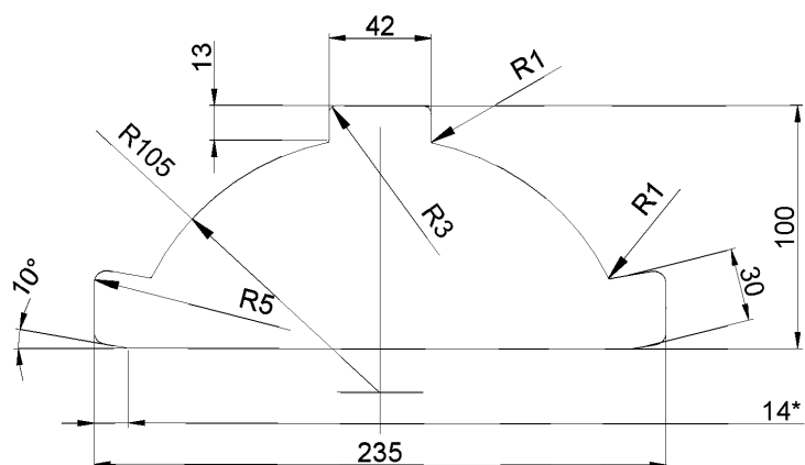
Рисунок Б.3 – Заглушка конька плоская (ЗКп)
