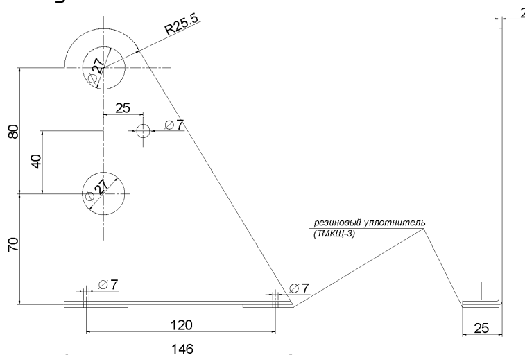
Рисунок Б.26 Кронштейн снегозадержателя 1 (КрСз/1)
