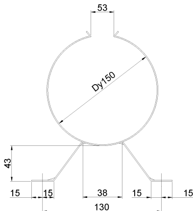
Рисунок Б.34 Держатель трубы 150 (ДТ150)
