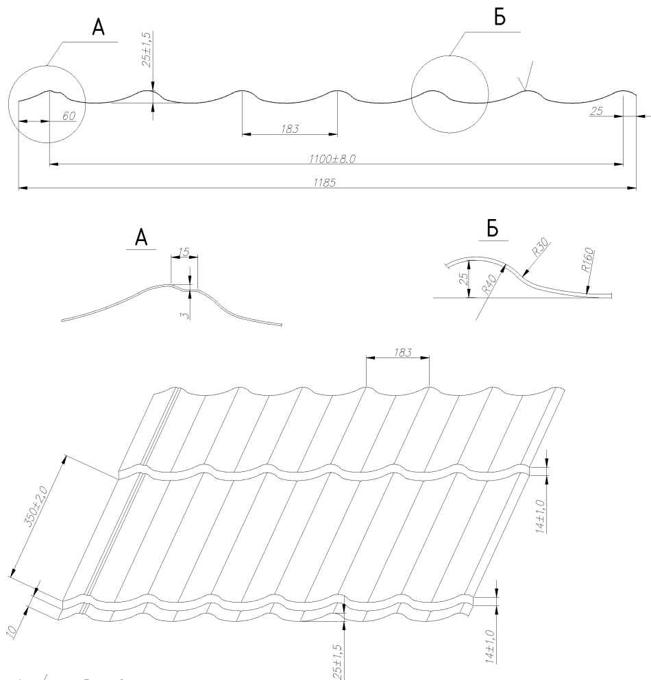
Рисунок 1 – металлочерепица «Monterrey» МЧ 39
