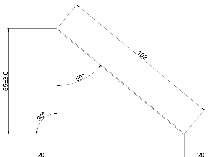
Рисунок Б.44 Планка снегозадержателя 2 (ПСз/2)
