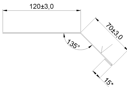
Рисунок Б.8 – Карниз (К)
