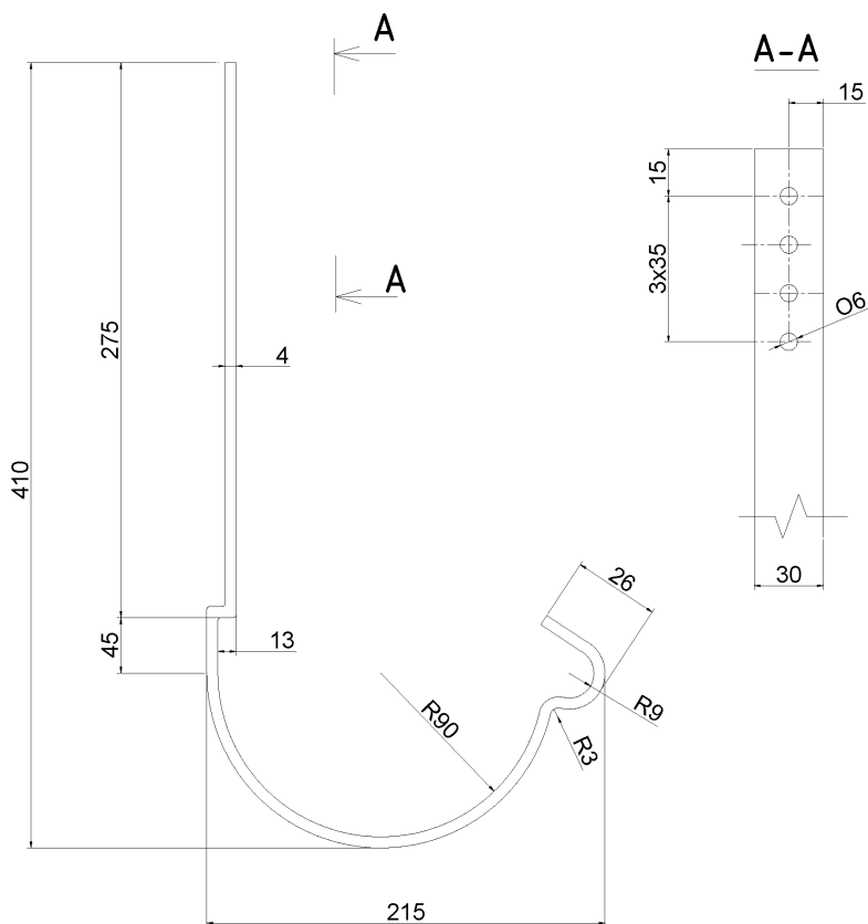
Рисунок Б.14 Держатель желоба 150 (Дж150)
