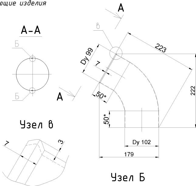
Рисунок Б.38 Колено сливное 100 (Ксл100)
