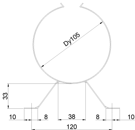
Рисунок Б.23 – Держатель трубы (ДТ100)
