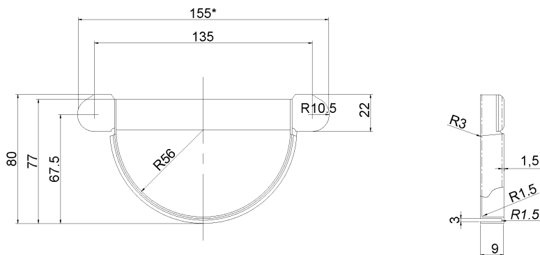
Рисунок Б.15 – Заглушка желоба (ЗЖ100)
