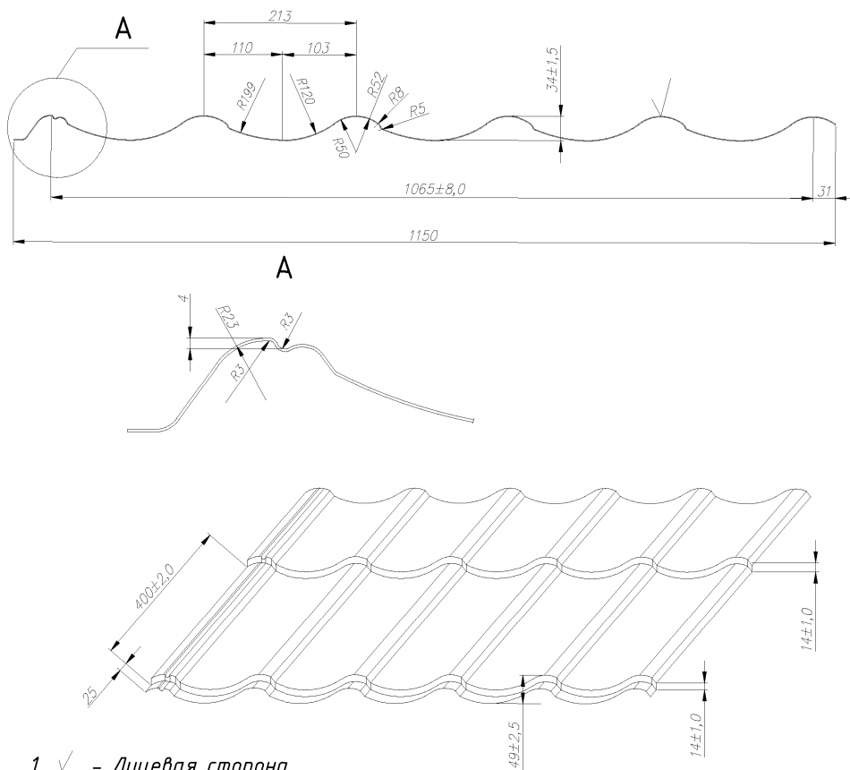
Рисунок 2 – металлочерепица «Joker» МЧ 49
