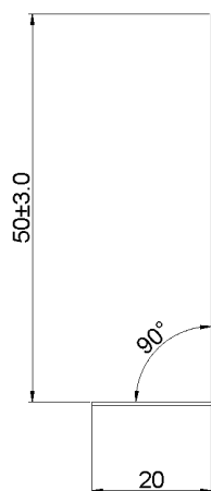
Рисунок Б.45 Усиление планки снегозадержателя 2 (УПСз/2)
