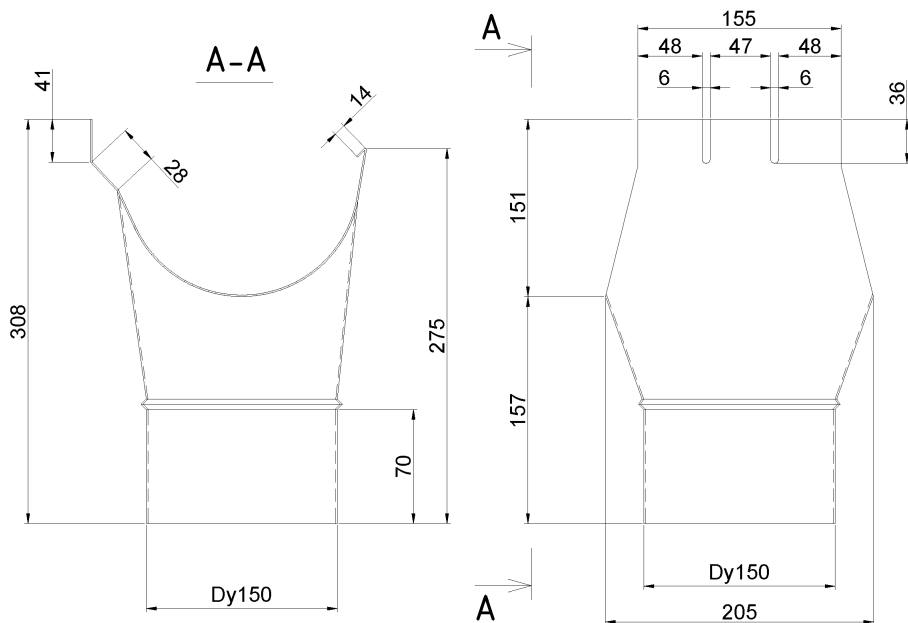
Рисунок Б.33 Патрубок 150 (П150)
