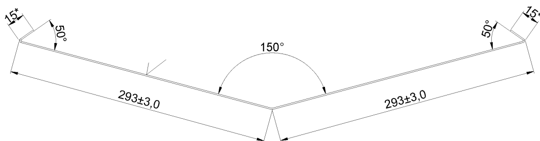
Рисунок Б.6 – Нижняя ендова (EH)
