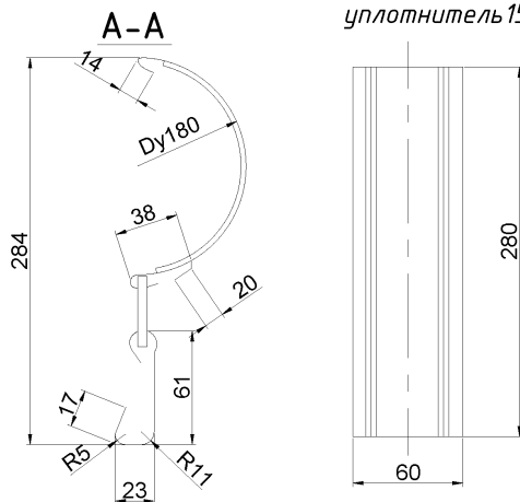
Рисунок Б.32 - Резиновый уплотнитель 150.
