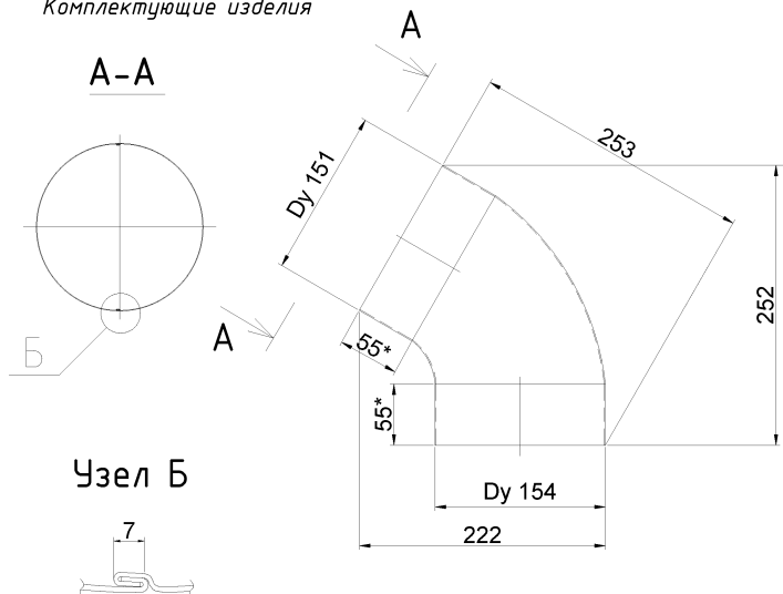
Рисунок Б.37 Колено угловое 150 (Куг150)
