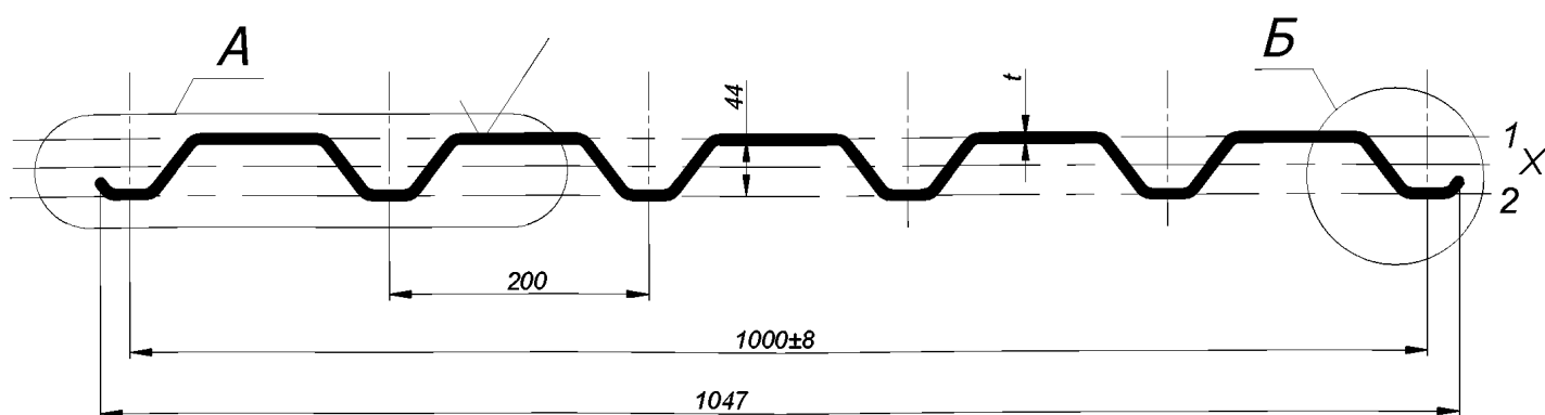
Рисунок 5.1 – Профилированный лист С44-1000 Вид1.
