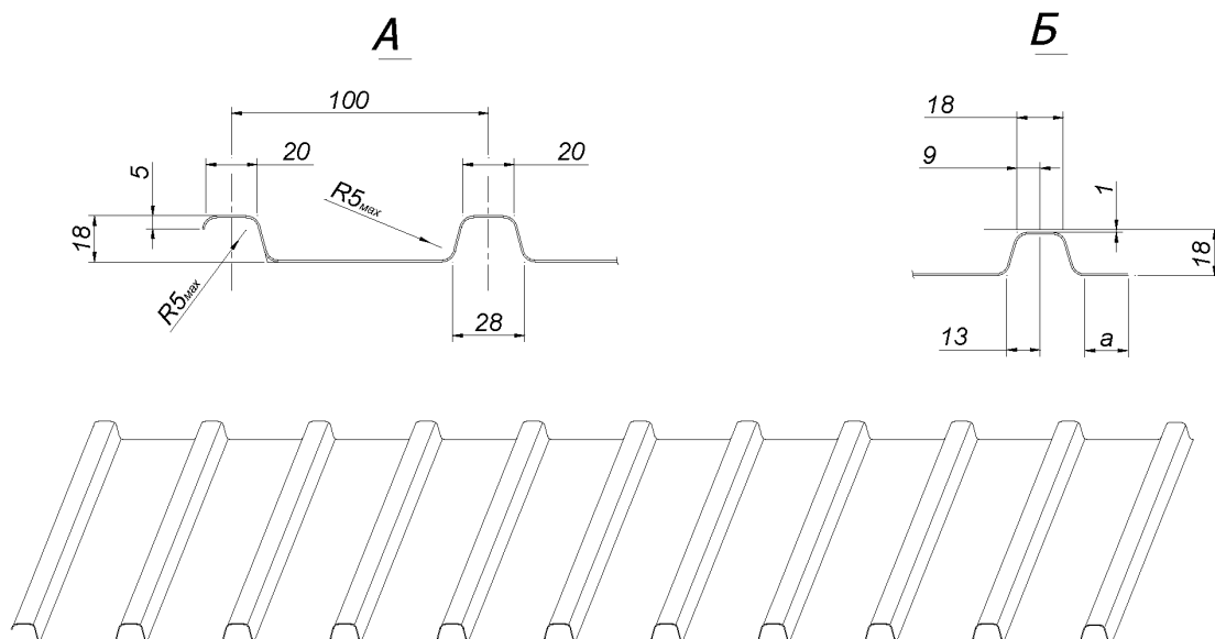
Рисунок 8 – Профилированный лист С18-1000.
