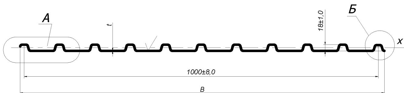
Рисунок 8 – Профилированный лист С18-1000.
