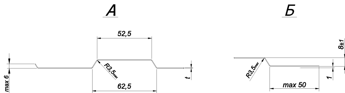
Рисунок 1 – Профилированный лист С8-1150
