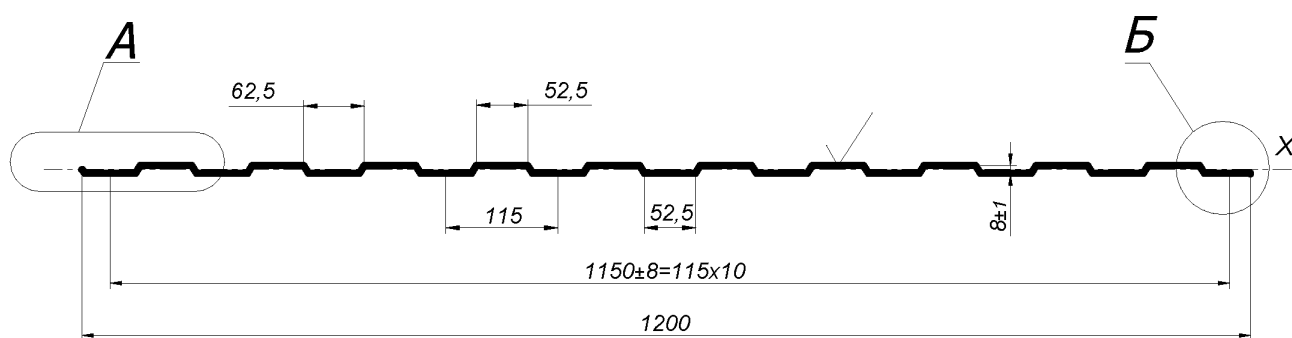
Рисунок 1 – Профилированный лист С8-1150
