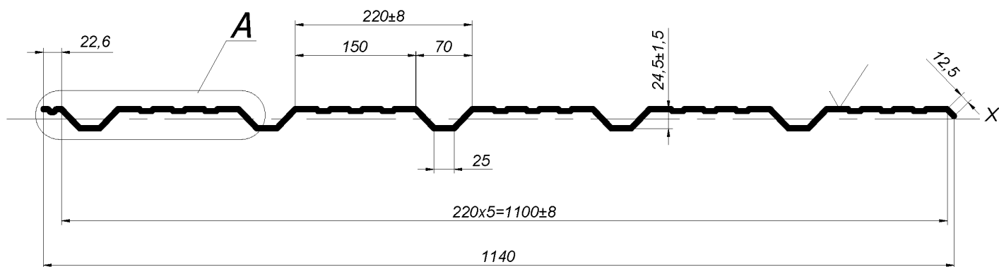
Рисунок 4.1 – Профилированный лист С25-1100. Вид 1
