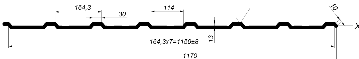
Рисунок 2.2 – Профилированный лист С13-А-1150 тип А. Вид 2
