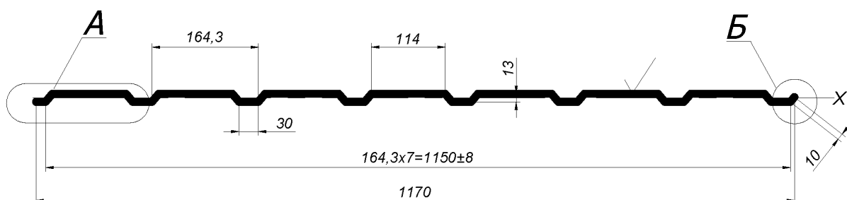
Рисунок 2.1 – Профилированный лист С13-А-1150 тип А. Вид 1
