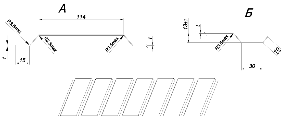
Рисунок 2.2 – Профилированный лист С13-А-1150 тип А. Вид 2
