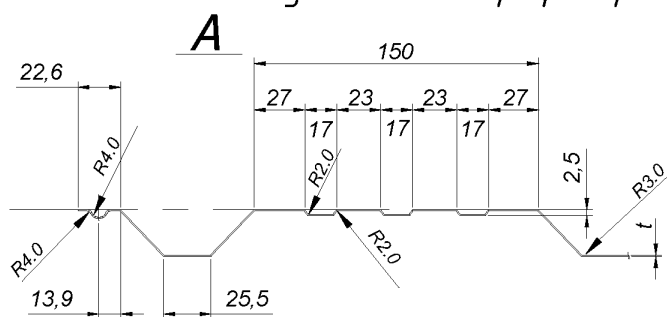
Рисунок 4.2 – Профилированный лист С25-1100. Вид 2
