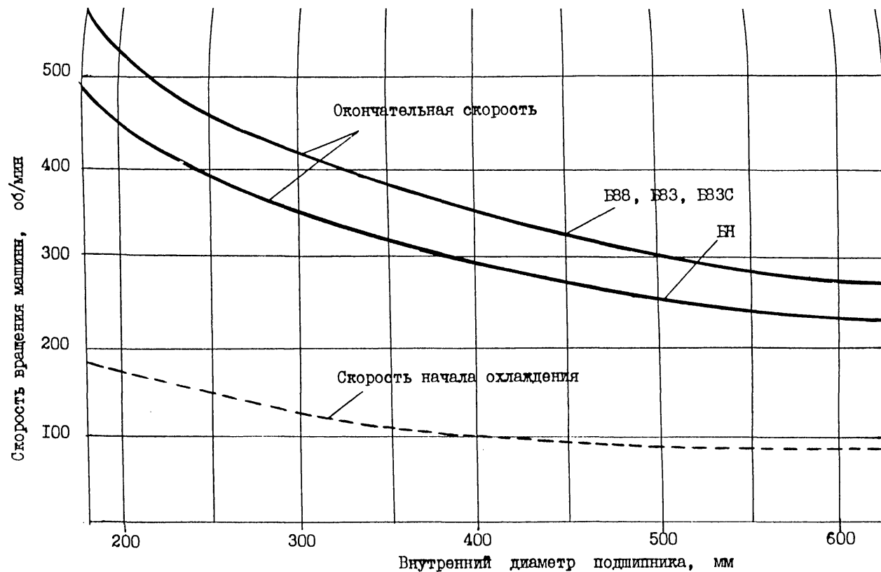
Рис. 3 Кривые для определения числа оборотов центробежной машины в зависимости от диаметра заливаемых подшипников
