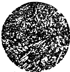
Рис. 3 Допустимая микроструктура. На фоне \alpha - фазы средне- и крупно- зернистые включения игольчатых кристаллов \gamma - фазы и участки ликвации.
