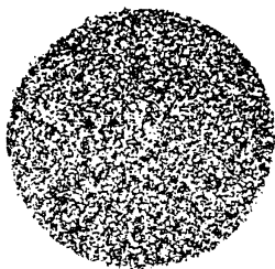
Рис. 12 Хорошая микроструктура Равномерное распределение от- носительно мелких кристаллов \beta -фазы в эвтектике \alpha(Pb) + \beta(SnSb)
