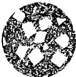
Рис. 6 Удовлетворительная микроструктура. Равномерное распределение кубовидных кристаллов \beta -фазы с размерами сторон 0,03-0,13 мм, игольчатых и звездчатых кристаллов \gamma -фазы
