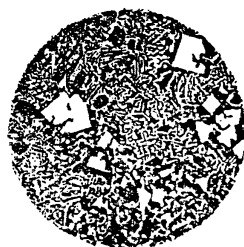
Рис. 13. Удовлетворительная микроструктура. Неравномерное распределение кристаллов \beta -фазы в эвтектике \alpha(Pb) + \beta(SnSb) при незна- чительной ликвации структурных составляющих
