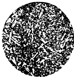
Рис. 2 Удовлетворительная микроструктура. На фоне \alpha - фазы среднезерни- стые включения игольчатых кристаллов \gamma - фазы.
