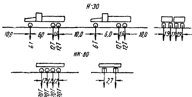
Рис. 3. Схема нормативных нагрузок
