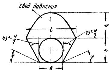
Рис. 2. Схема свода давления
