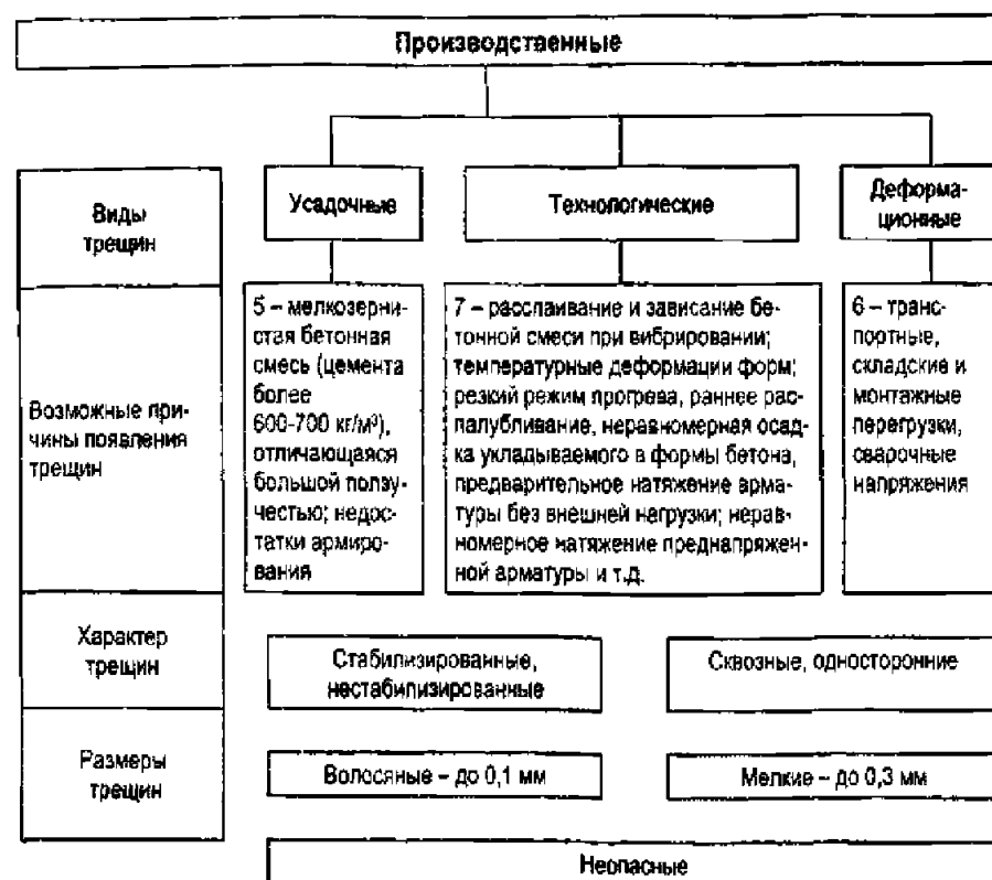
Рисунок Г.1 – Классификация трещин в железобетонных конструкциях
