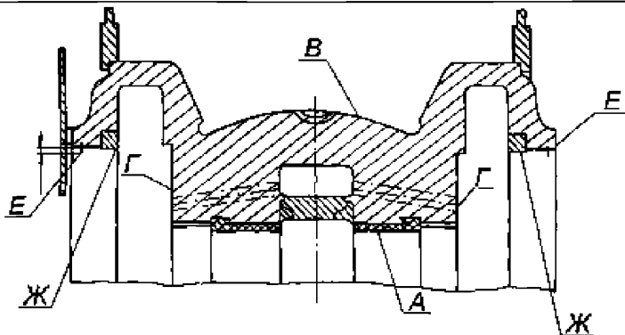
Карта дефектации и ремонта 18 Вкладыш опорно-упорного подшипника, поз. 3 рисунок 7.5 Количество на изделие, шт. – 1
