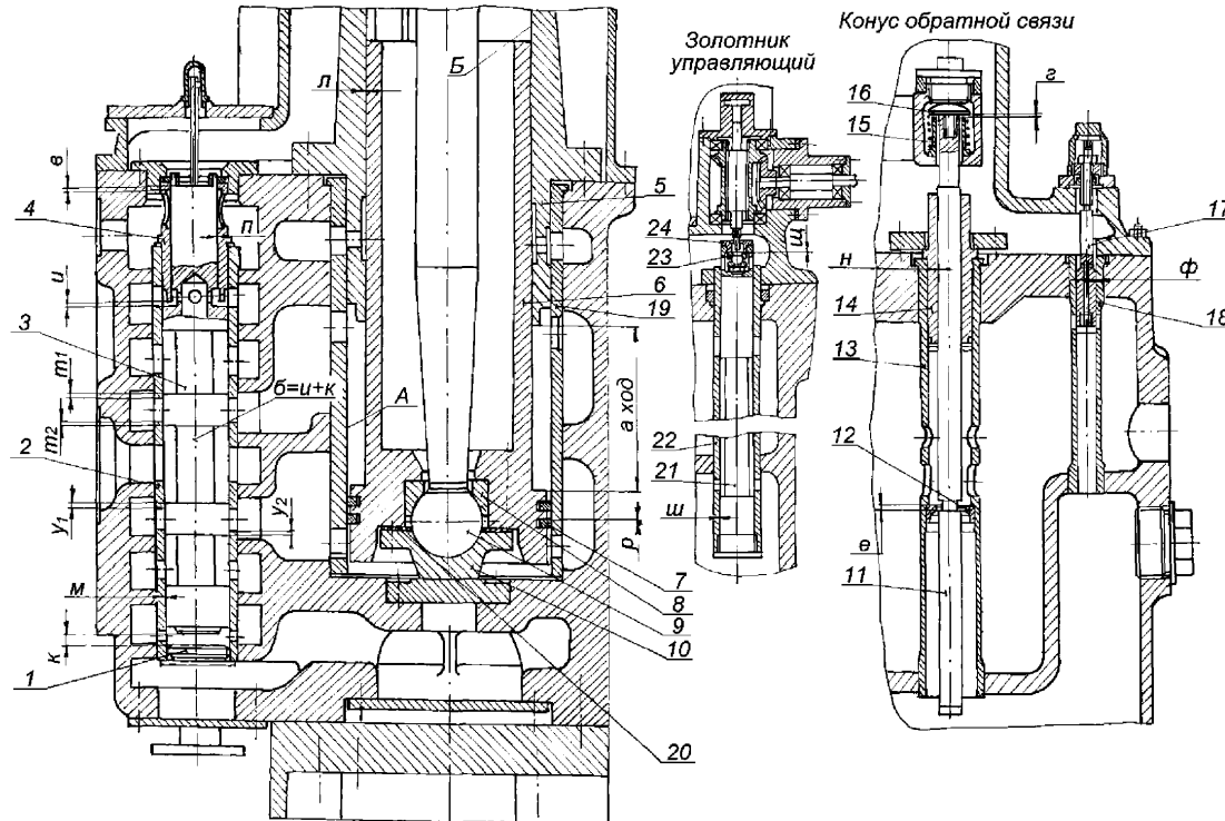
Рисунок 7.24 – Сервомотор ЧСД
