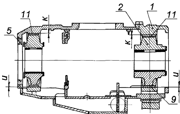
Рисунок 7.6 – Подшипники № 4–5
