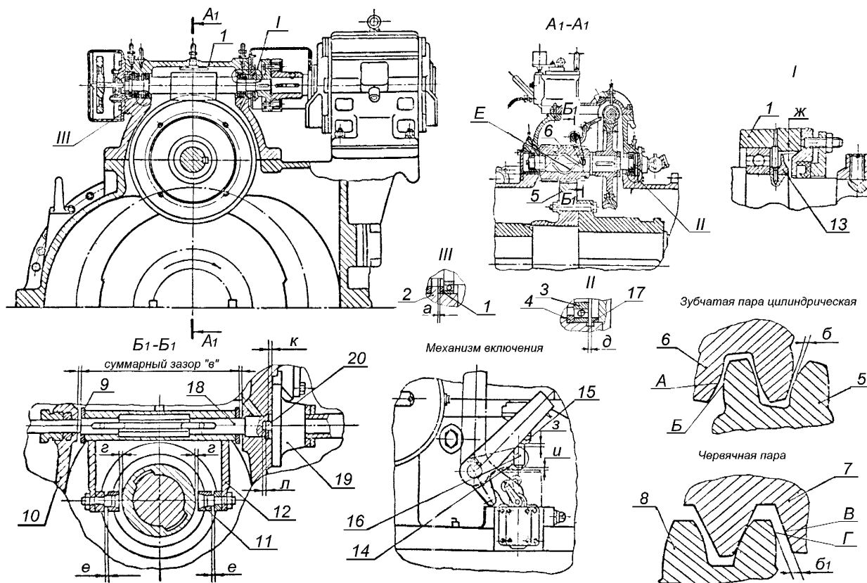
Рисунок 7.7 – Валооборотное устройство
