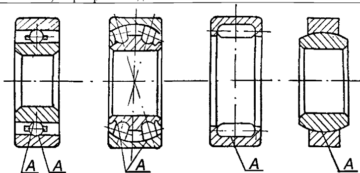
Карта дефектации и ремонта 34 Подшипники качения, шарнирные подшипники
