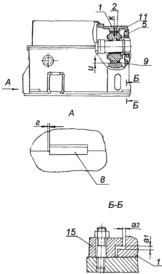
Рисунок 7.4 – Передний подшипник
