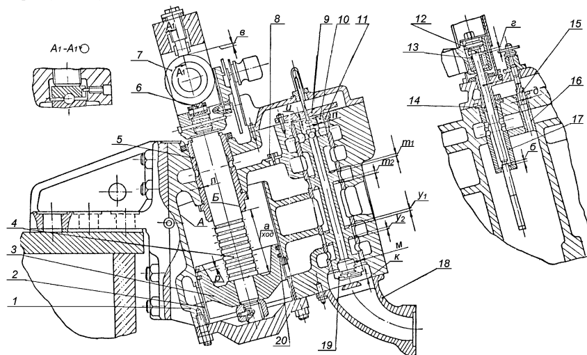
Рисунок 7.27 – Сервомотор ЧНД
