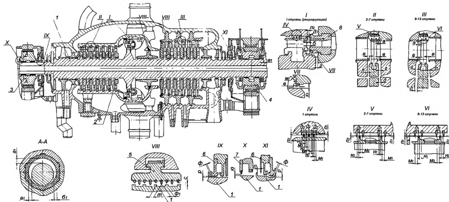
Рисунок 7.8 – Цилиндр ВД
