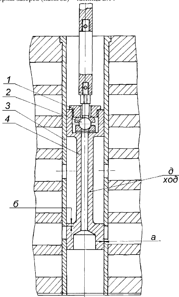
Рисунок 7.17 – Выключатель РД
