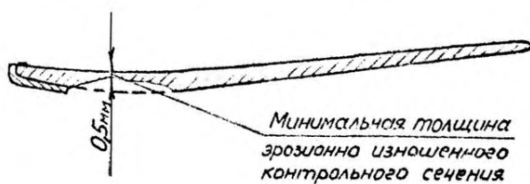
Рисунок Д.4.1 – Измерение эрозионного износа рабочих лопаток 25 (28) ступе- ни
