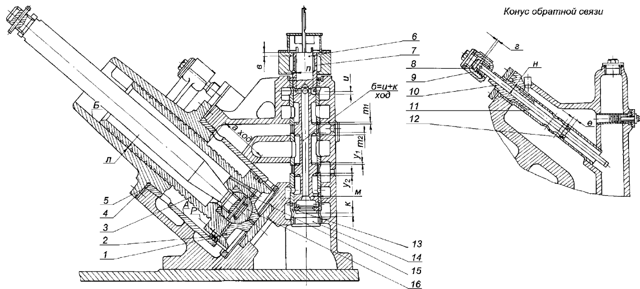
Рисунок 7.23 – Сервомотор ЧВД
