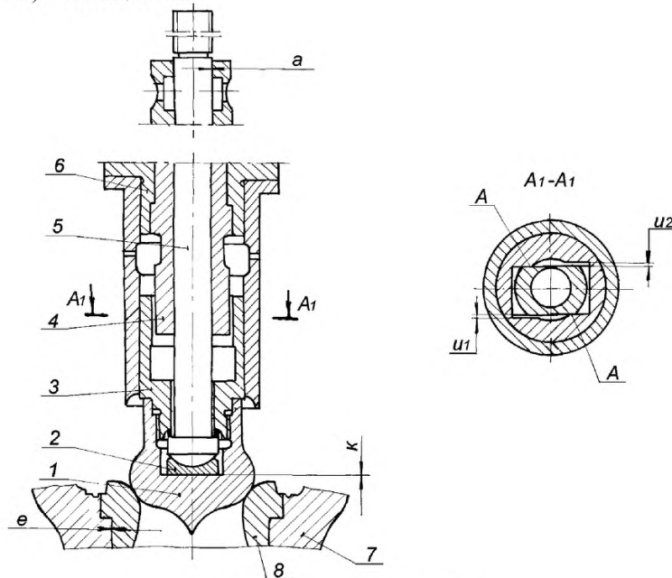
Рисунок 7.35 – Клапаны регулирующие ЧСД
