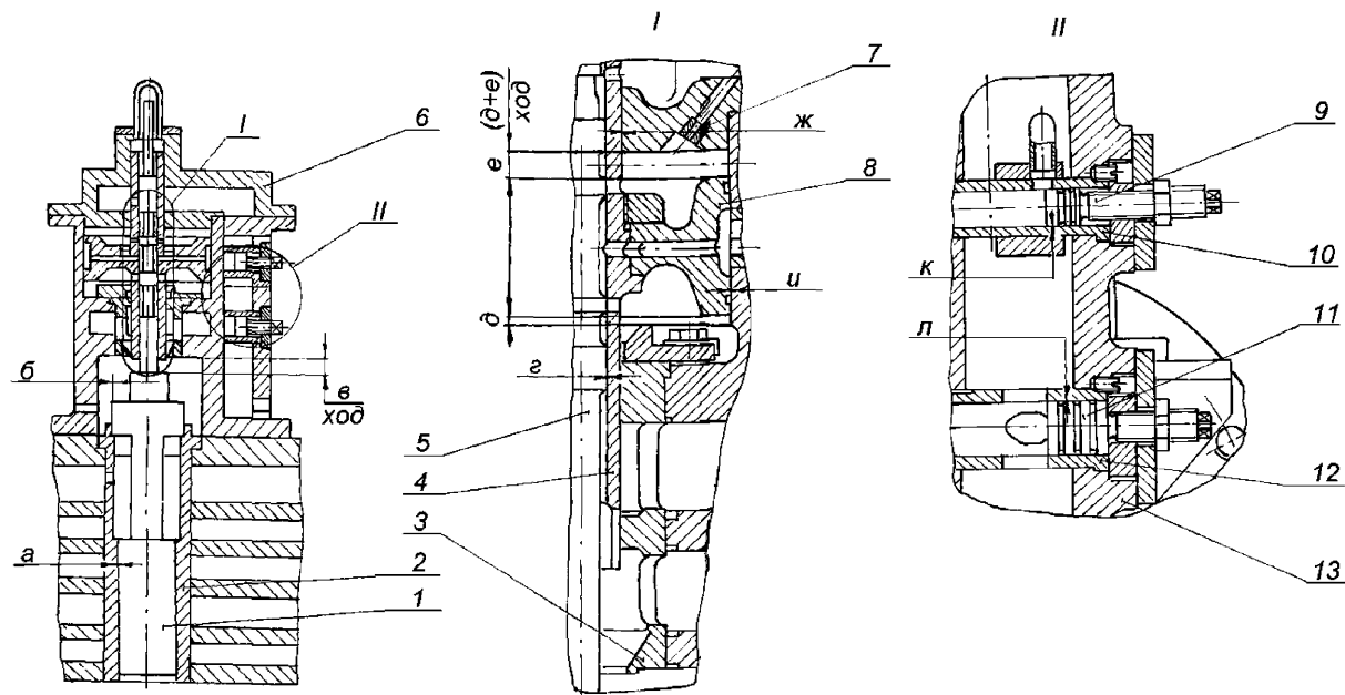
Зазоры a , b , г , ж , и , к , л заданы на диаметр Рисунок 7.15 – Регулятор давления ПО и нижнего ТО
