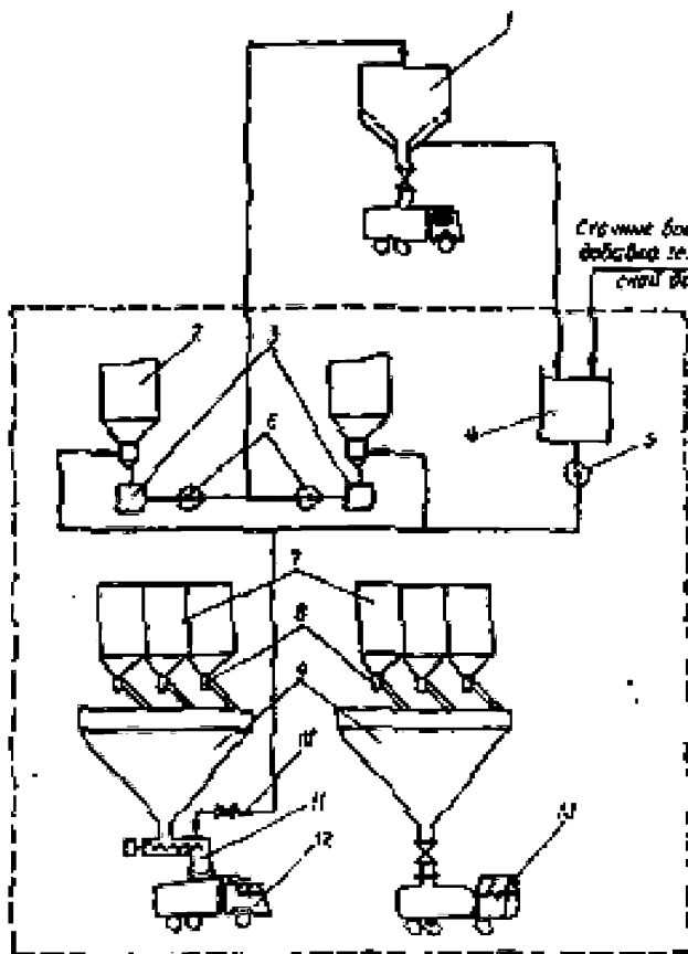
Такая схема рекомендуется, если потребность в сухой золе все время или в отдельные периоды работы ТЭС будет меньше, чем количество золы, улавливаемой золоуловителями. Если потребляется вся зола или применяется метод сухого складирования летучей золы, целесообразно применять схему, приведенную на рисунке А.10.
