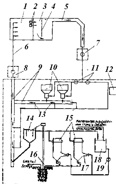
Рисунок А.4 – Схема гидрозолоудаления ТЭС оборудованной мокрыми золоуловителями с автономным циклом орошения
