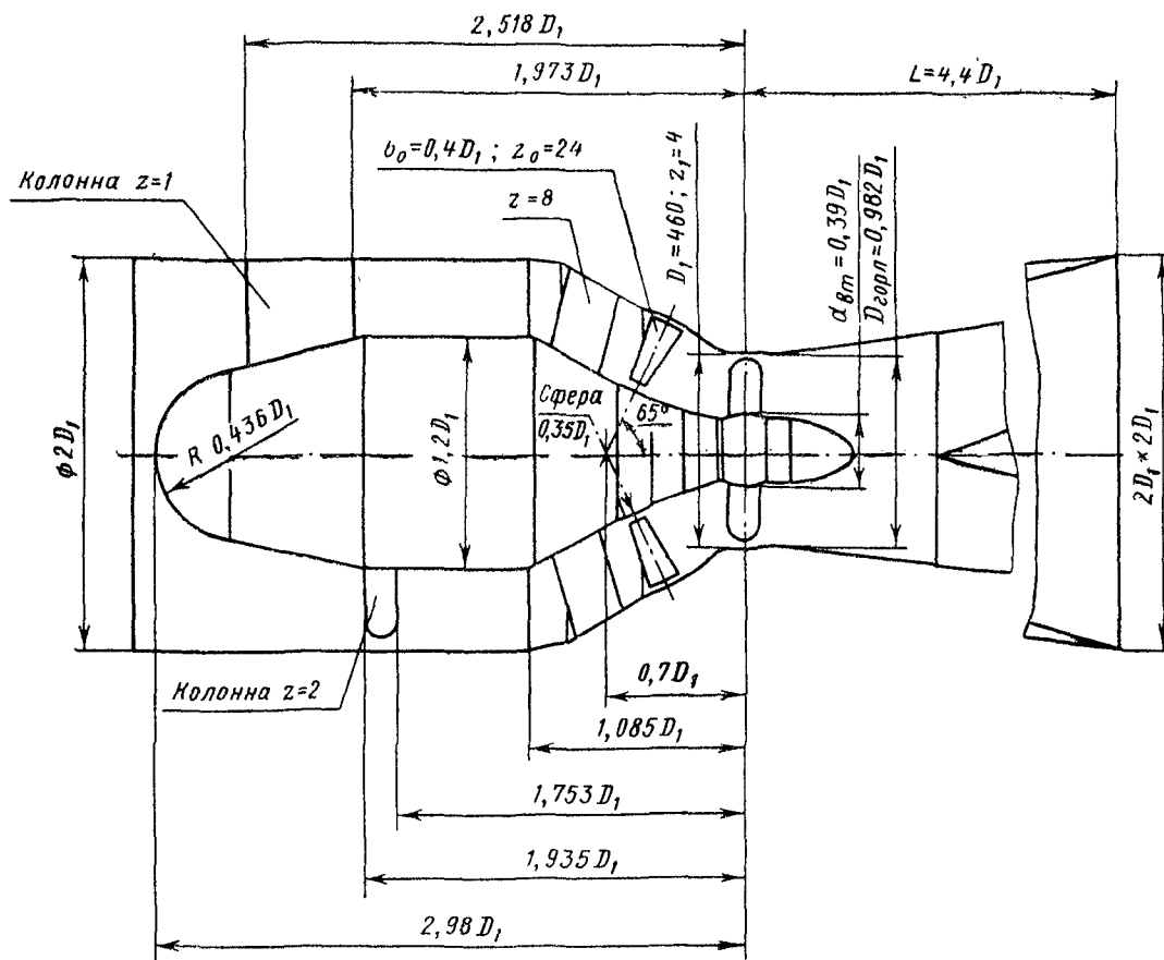
Проточная часть модели гидротурбины ПЛ 25/3161-ГК-46 (к универсальной характеристике № 2572 ХТГЗ)
