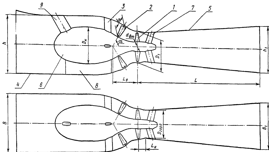
Проточная часть капсульной гидротурбины с выходным статором
