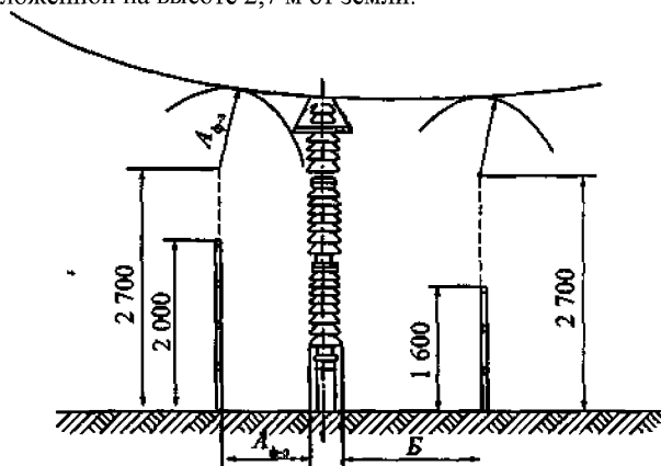
Рисунок 3 - Схема размещения оборудования. Наименьшие расстояния от токоведущих частей и элементов изоляции, находящихся под напряжением, до постоянных внутренних ограждений
