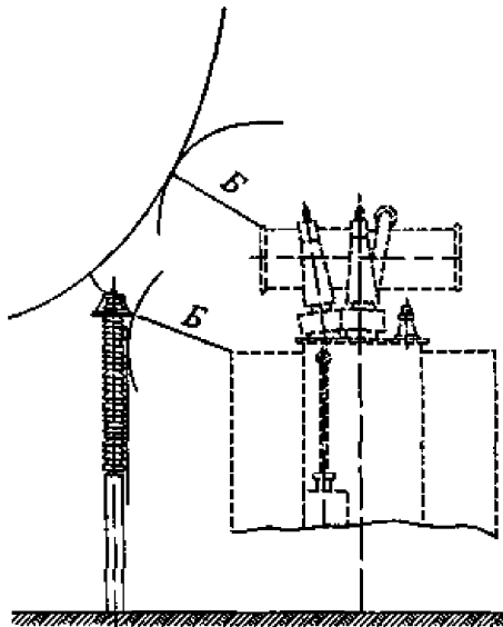
Рисунок 5 - Схема размещения оборудования. Наименьшие расстояния от токоведущих частей до транспортируемого оборудования
