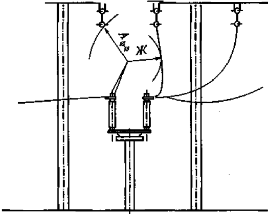
Рисунок 9 - Схема размещения оборудования. Наименьшие расстояния от подвижных контактов разъединителей в отключенном положении до заземленных и токоведущих частей
