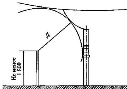
Рисунок 8 - Схема размещения токоведущих частей. Наименьшие расстояния от токоведущих частей до верхней кромки внешнего ограждения
