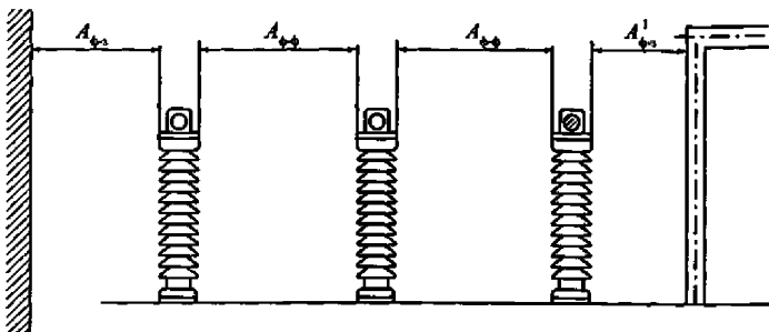
Рисунок 1 – Схема размещения оборудования. Наименьшие расстояния в свету при жестких шинах между токоведущими и заземленными частями ( A_{\phi-3} , A'_{\phi-3} ) и между токоведущими частями разных фаз ( A_{\phi-\phi} )
