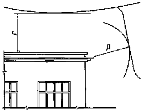
Рисунок 10 - Схема размещения токоведущих частей. Наименьшие расстояния между токоведущими частями и зданиями и сооружениями
