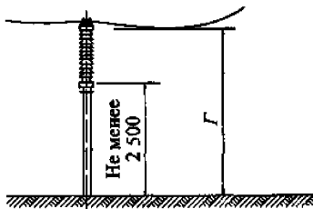
Рисунок 4 - Схема размещения оборудования. Наименьшие расстояния от не огражденных токоведущих частей и от нижней кромки фарфора изоляторов до земли
