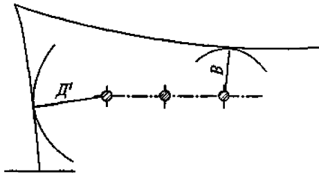
Рисунок 6 - Схема размещения токоведущих частей. Наименьшие расстояния между токоведущими частями разных цепей, расположенными в различных плоскостях с обслуживанием нижней цепи при не отключенной верхней
