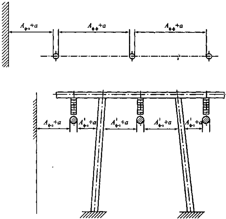
Рисунок 2 – Схема размещения оборудования. Наименьшие расстояния в свету при гибких шинах между токоведущими и заземленными частями и между токоведущими частями разных фаз, расположенными в одной горизонтальной плоскости
