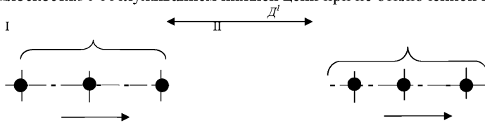
Рисунок 7 - Схема размещения токоведущих частей. Наименьшие расстояния по горизонтали между токоведущими частями разных цепей с обслуживанием одной цепи при неотключенной другой
