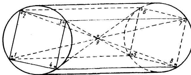
Схема размещения в камере датчиков температуры (влажности)
