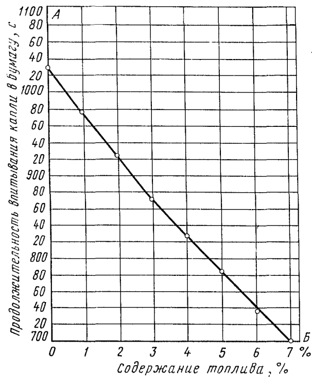
Рис. 8. Зависимость скорости впитывания капли от содержания топлива до 7 и 15% в смазочном масле
