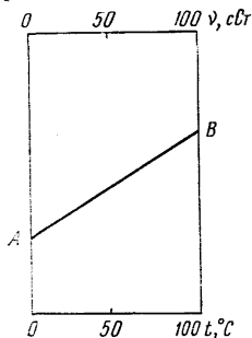
Рис. 9. Номограмма для уравнения Вальтера:
