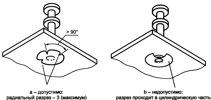
Рисунок 2 — Разрывы развальцованного фланца, обжатого роликом
