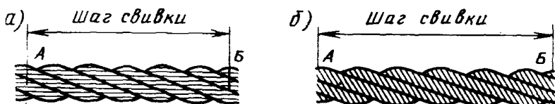
Канаты для грузоподъемных машин: а — крестовой свивки; б — односторонней свивки
