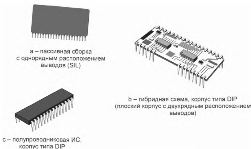
Рисунок 12 — Типовые конструктивные исполнения многвыводных корпусов ИС
