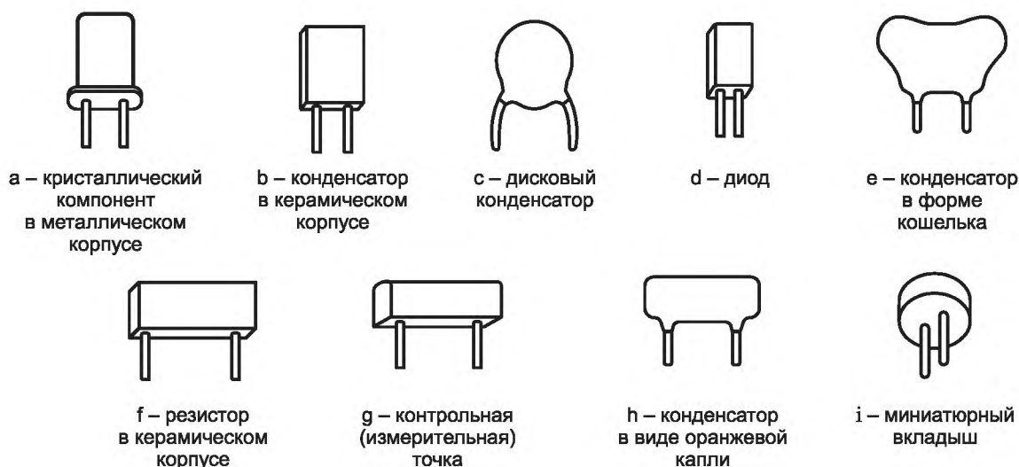
Рисунок 9 — Типовые компоненты с двумя радиальными выводами
