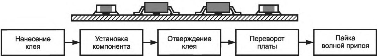
Рисунок 2 — Односторонний печатный узел. Пайка только погружением
