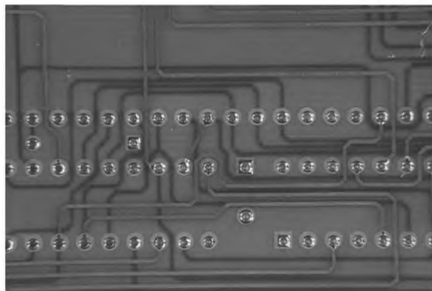
Рисунок 11 — Паяльная маска: допустимое состояние
