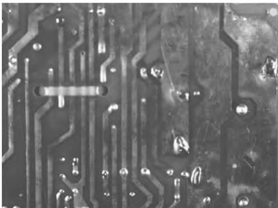
Рисунок 77 — Остатки флюсов: недопустимое состояние
