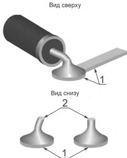
Рисунок 72 — Обнажение основного металла: допустимое состояние
