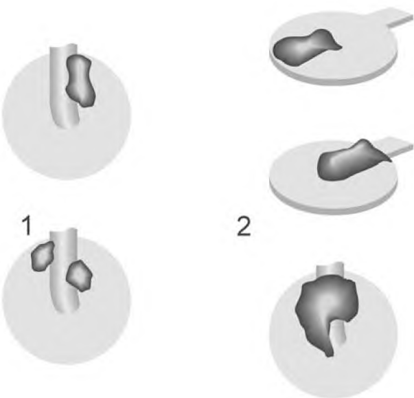
Рисунок 70 — Загнутые выводы, неметаллизированные сквозные отверстия: допустимое состояние
