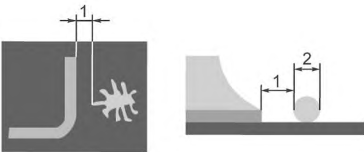
Рисунок 59 — Шарики или бусинки припоя: недопустимое состояние
