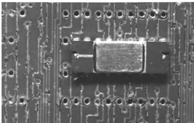
Рисунок 12 — Паяльная маска, растрескивание или вздутие: виды состояний
