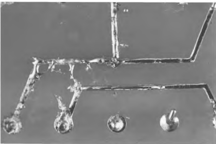
Рисунок 60 — Перемычки припоя: недопустимое состояние
