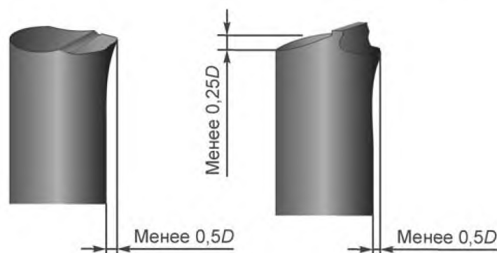
Рисунок 9 — Обрезка вывода: допустимое состояние
