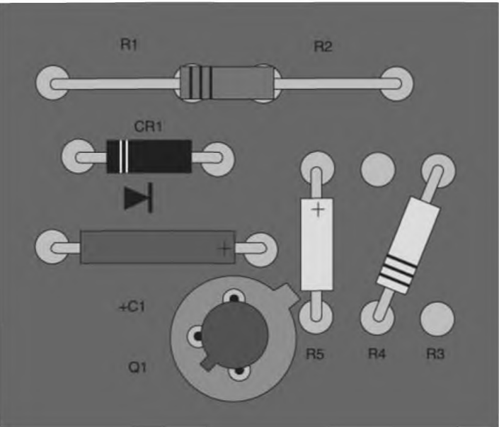
Рисунок 19 — Ориентация компонента: недопустимое состояние
