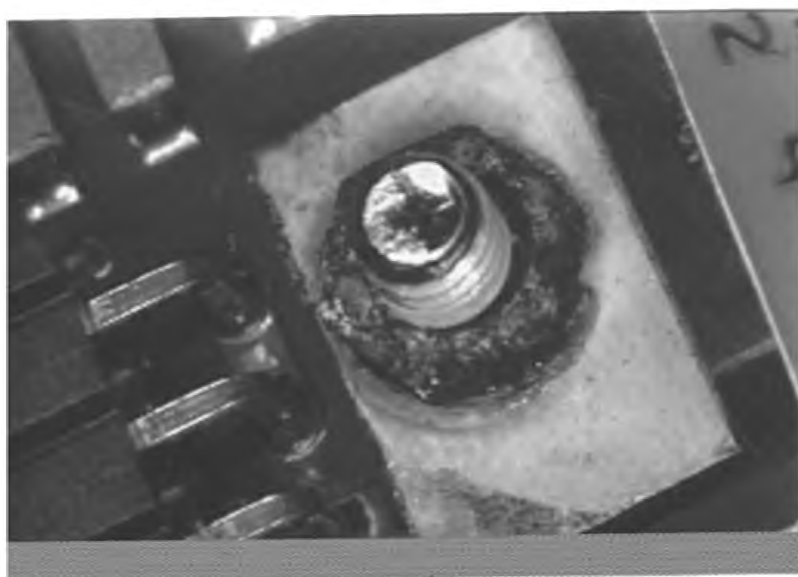
Рисунок 84 — Остатки коррозии на деталях: недопустимое состояние
