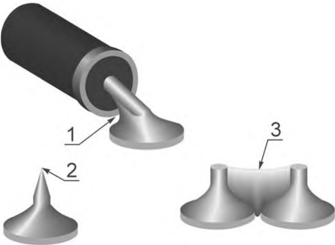
Рисунок 69 — Паяное соединение: недопустимое состояние
