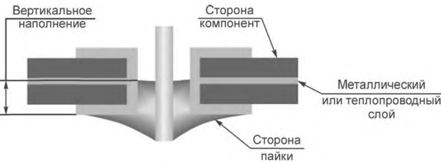
Рисунок 64 — Тепловой слой, наполнение отверстия припоем: виды состояний
