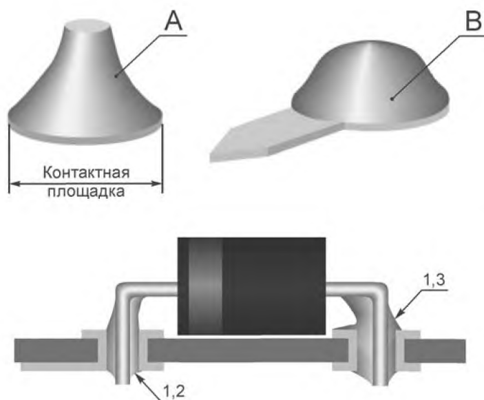
Рисунок 62 — Смачивание припоем: допустимое состояние
