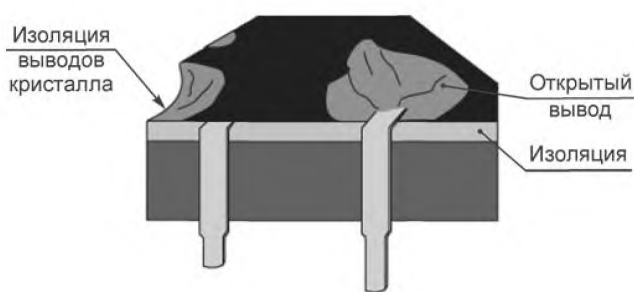
Рисунок 54 — DIP-корпус: недопустимое состояние
