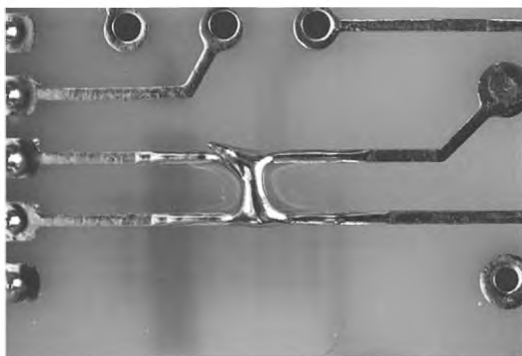
Рисунок 57 — Избыток припоя, образование перемычек: недопустимое состояние
