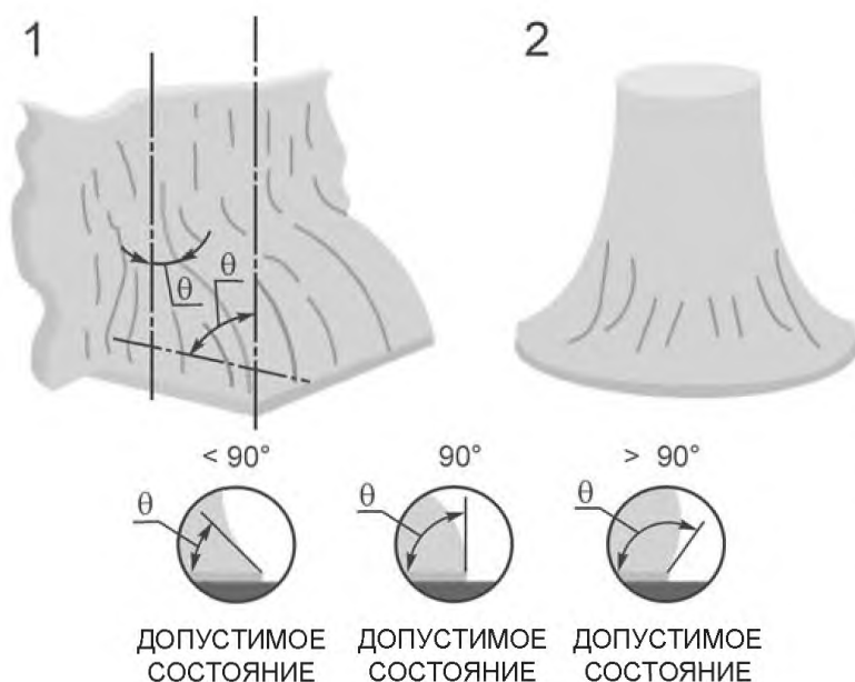
Рисунок 55 — Паяные соединения в сквозные отверстия: допустимое состояние
