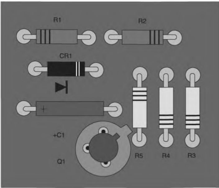
Рисунок 18 — Ориентация компонента: допустимое состояние
