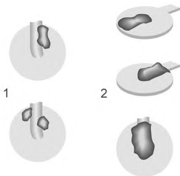
Рисунок 71 — Загнутые выводы, металлизированные сквозные отверстия: допустимое состояние
