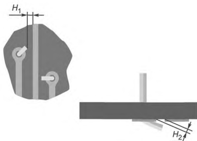
Рисунок 6 — Частично загнутый вывод: допустимое состояние
