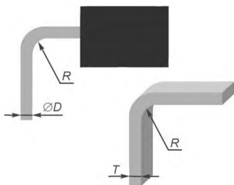
Рисунок 2 — Изгиб вывода: допустимое состояние
