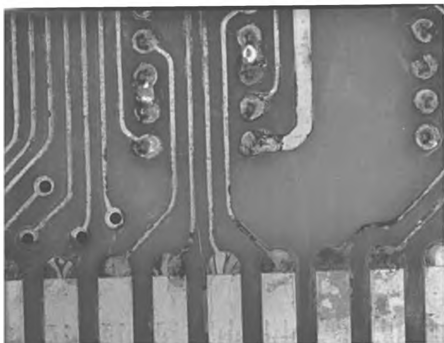
Рисунок 85 — Остатки коррозии на печатной плате: недопустимое состояние
