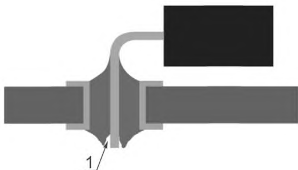
Рисунок 75 — Разрывы в контакте: недопустимое состояние
