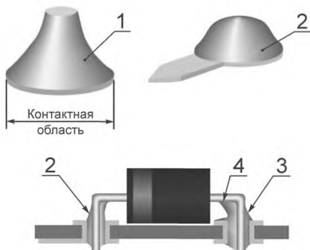
Рисунок 66 — Галтель припоя: допустимое состояние
