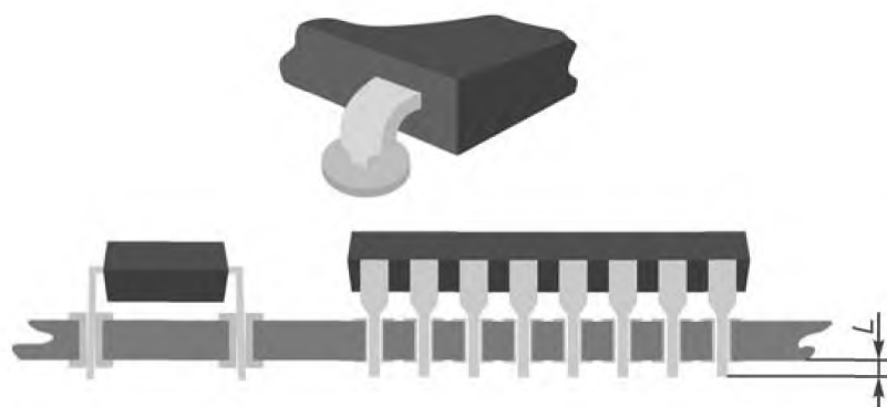
Рисунок 31 — Корпуса DIP: заданное состояние
