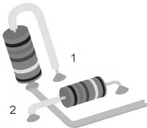
Рисунок 40 — Выводы, пересекающие проводники: допустимое состояние
