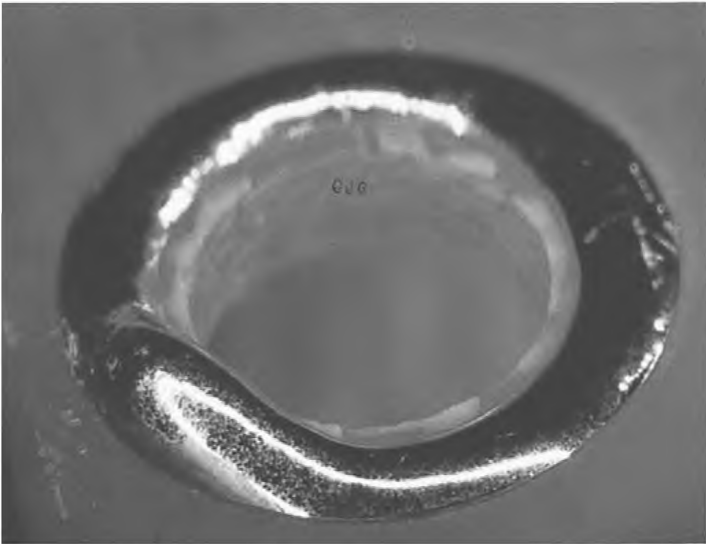
Рисунок 58 — Избыток припоя на монтажном отверстии: недопустимое состояние
