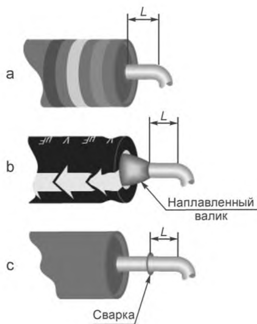
Рисунок 1 — Длина вывода до изгиба: допустимое состояние
