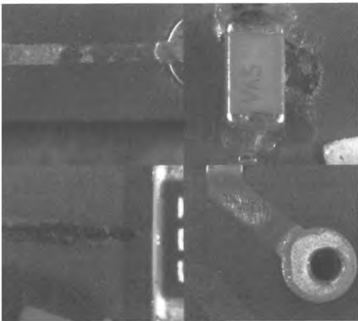
Рисунок 16 — Ухудшение физических параметров паяльной маски: недопустимое состояние
