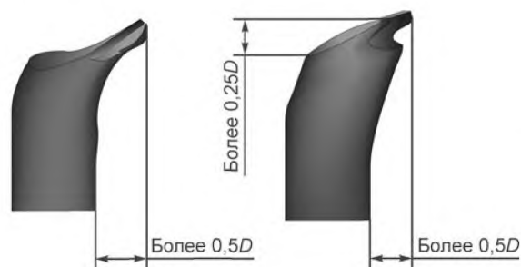
Рисунок 10 — Обрезка вывода: недопустимое состояние
