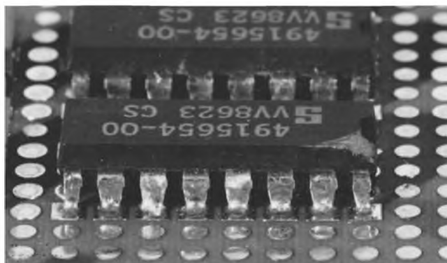
Рисунок 53 — DIP-корпус: допустимое состояние
