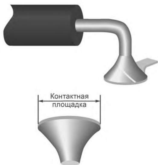
Рисунок 61 — Смачивание припоем: заданное состояние
