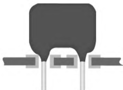
Рисунок 38 — Мениски покрытия, углубленные в отверстия: допустимое состояние
