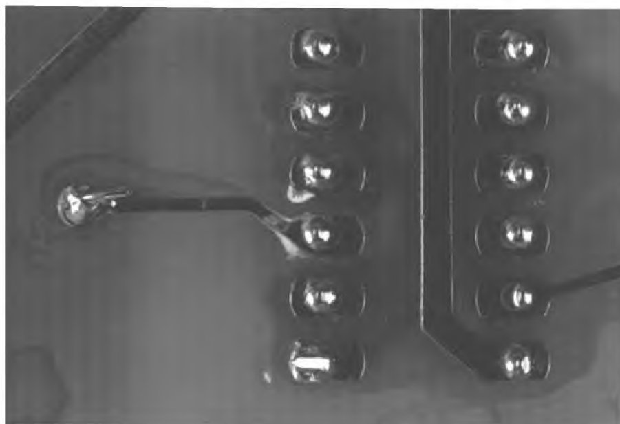
Рисунок 81 — Белесые остатки: недопустимое состояние
