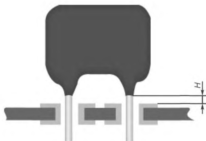
Рисунок 37 — Мениск покрытия над отверстием: заданное состояние
