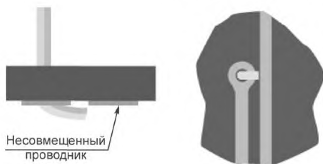
Рисунок 7 — Загнутый вывод: недопустимое состояние
