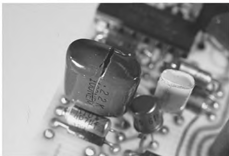
Рисунок 51 — Структурная целостность активной области: недопустимое состояние
