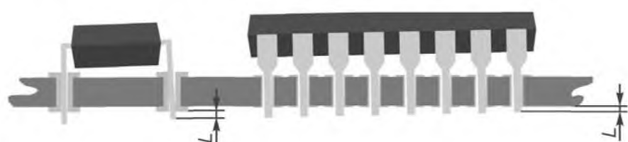
Рисунок 32 — Корпуса DIP: допустимое состояние
