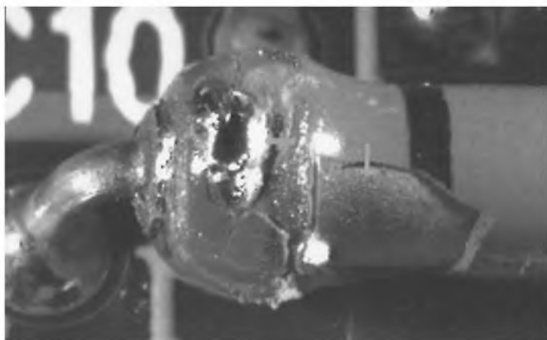
Рисунок 47 — Повреждение корпуса компонента с осевыми выводами: недопустимое состояние
