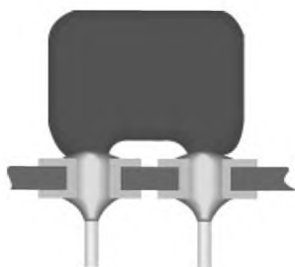
Рисунок 39 — Мениски покрытия, углубленные в отверстия: недопустимое состояние
