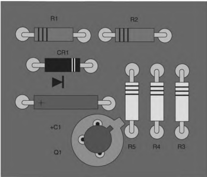
Рисунок 17 — Ориентация компонента: заданное состояние
