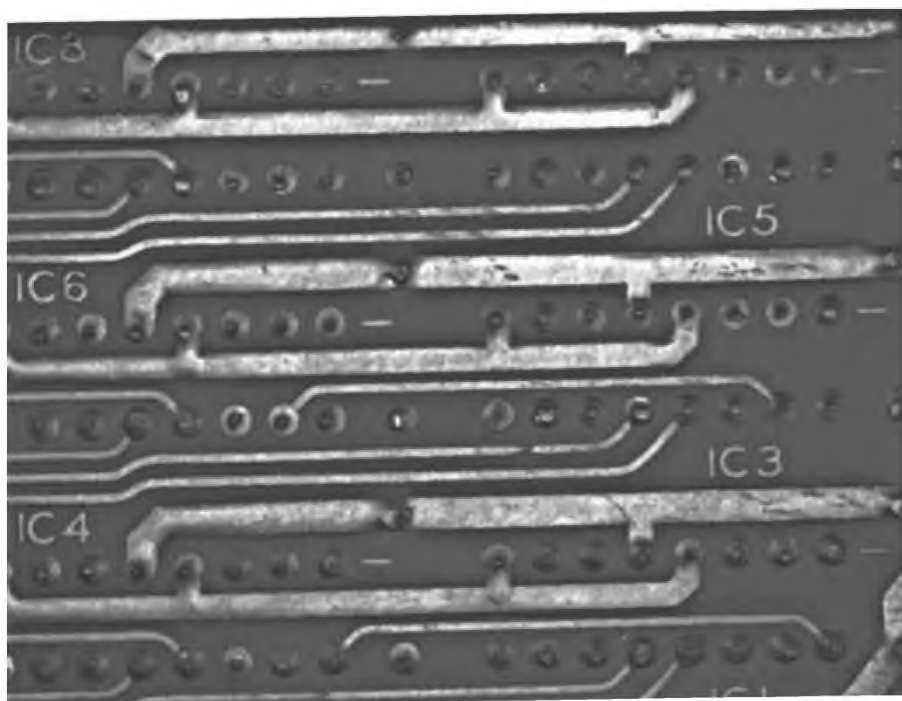
Рисунок 83 — Остатки коррозии: допустимое состояние
