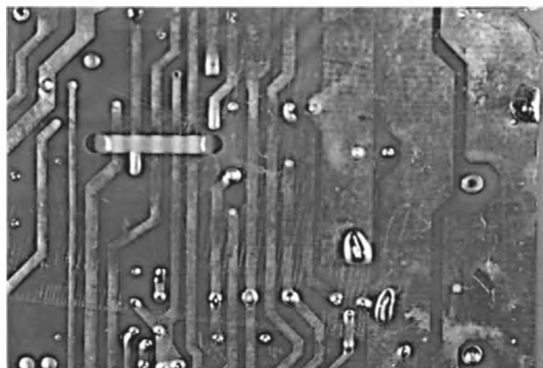
Рисунок 76 — Очистка: допустимое состояние
