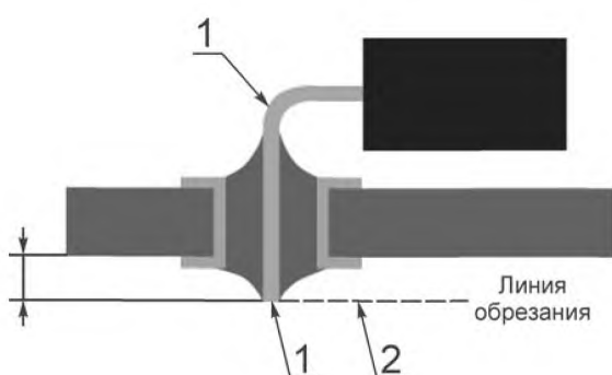
Рисунок 74 — Обрезанные выводы: допустимое состояние
