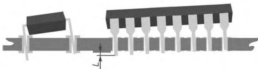
Рисунок 33 — Корпуса DIP: недопустимое состояние
