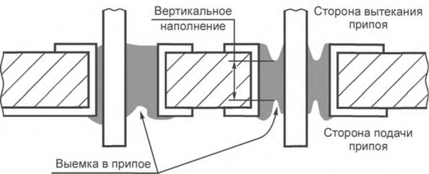
Рисунок 63 — Конфигурация заполнения отверстия и вывода: допустимое состояние
