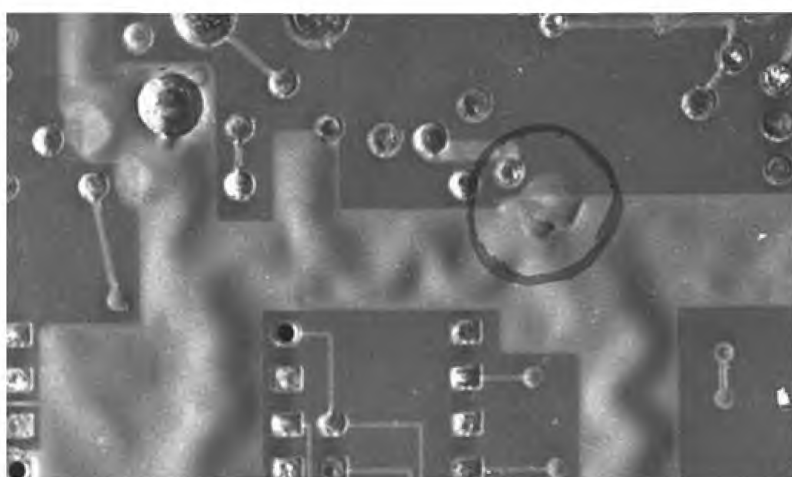
Рисунок 13 — Паяльная маска, свободные частицы: недопустимое состояние
