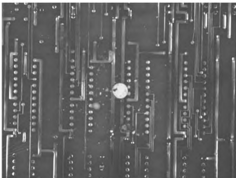
Рисунок 79 — Остатки в виде твердых частиц: недопустимое состояние
