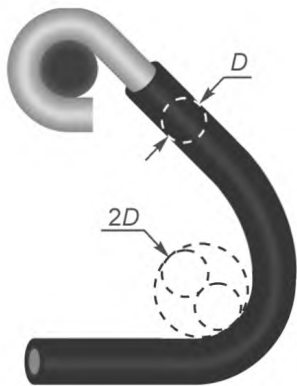
Рисунок 11 — Снятие напряжения с проволочного вывода: допустимое состояние
