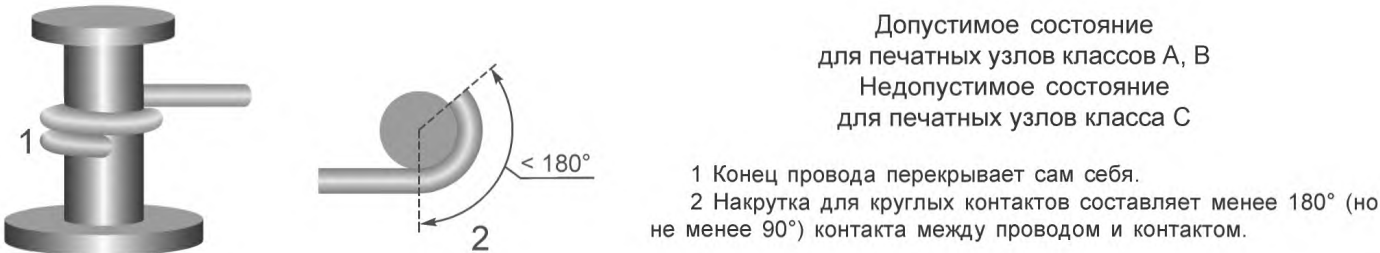
Рисунок 4 — Круговая накрутка провода и вывода: виды состояний
