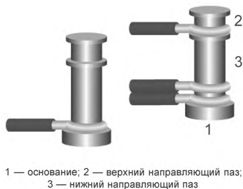
Рисунок 3 — Круговая накрутка провода и вывода: допустимое состояние
