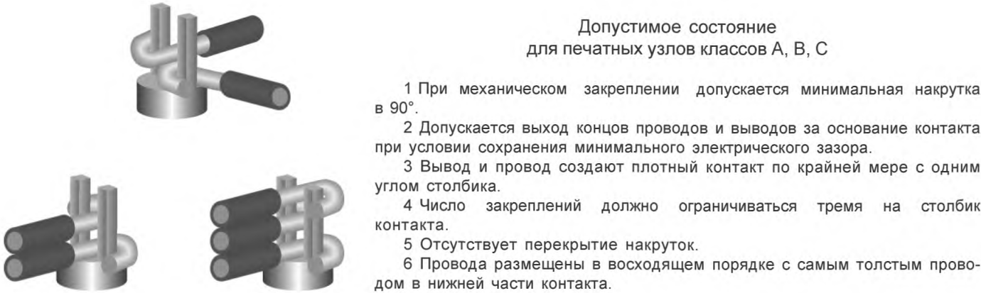
Рисунок 6 — Боковое соединение разводки, вилкообразный контакт: допустимое состояние
