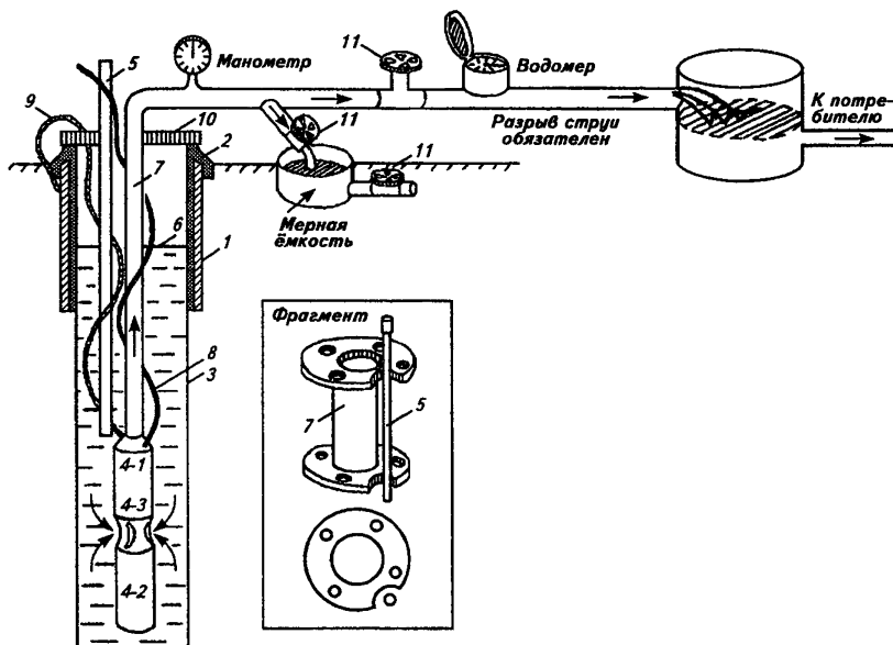
Схема оборудования эксплуатационной скважины на воду
