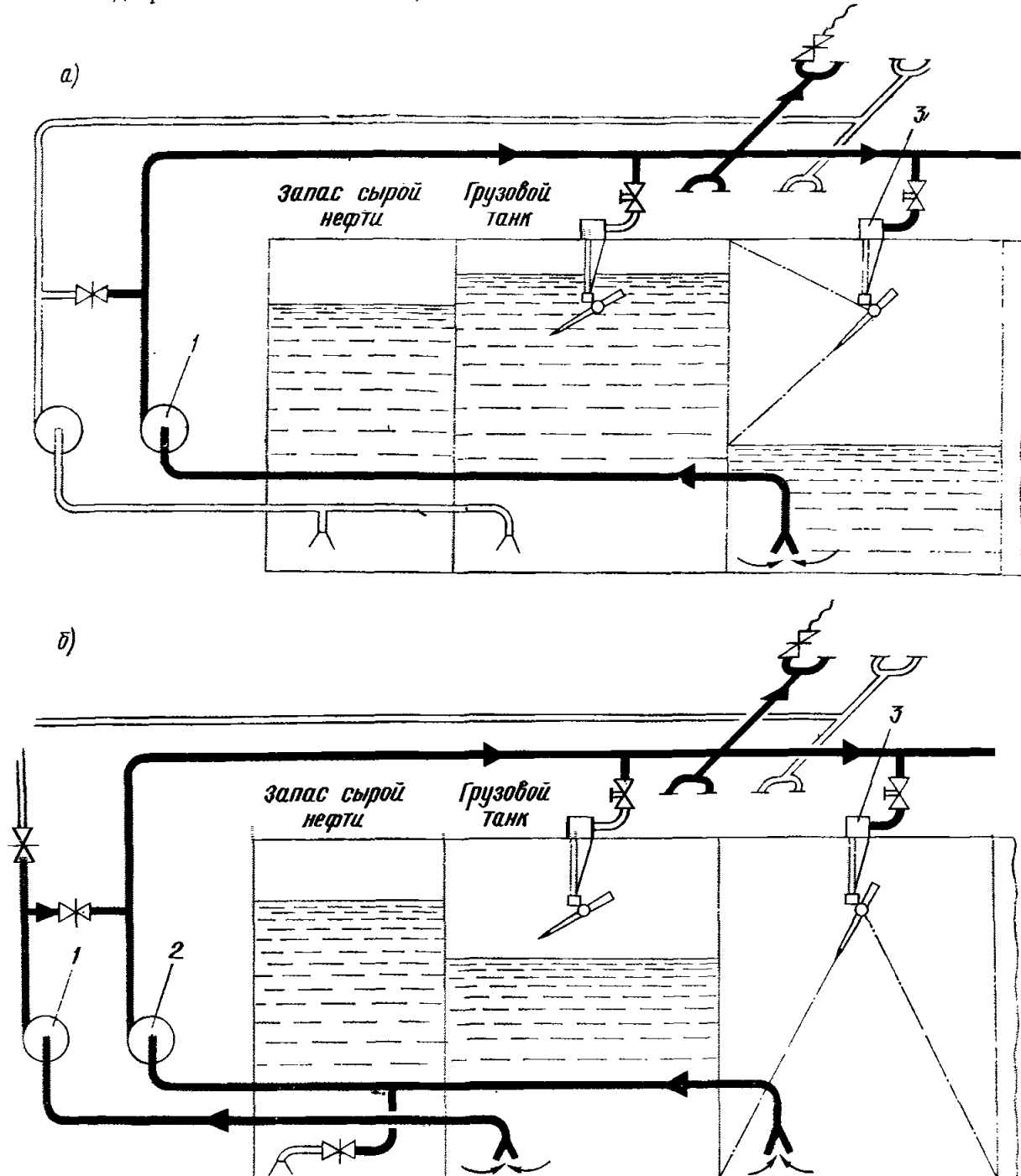
Рис. 5. Типовая схема мойки танков грузом сырой нефти двухэтапным способом: а — 1-й этап — мойка переборок; б — 2-й этап — мойка днища; 1 — грузовой насос, используемый для зачистки; 2 — зачистной насос; 3 — стационарная моечная машинка
