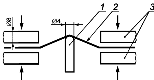
1 — оправка, например, шпиндельная наставка со стальным шариком; 2 — испытываемый образец; 3 — приспособление для крепления образца
