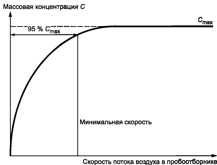
Рисунок 1 — Типичная зависимость массовой концентрации, полученной с помощью диффузионных пробоотборников, от скорости потока воздуха
