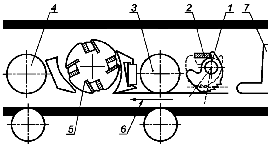
1 — устройство противоотдачи из качающихся планок; 2 — стопор для качающейся планки; 3 — приводной подающий ролик на входе; 4 — приводной подающий ролик на выходе; 5 — ножевой вал; 6 — направление подачи; 7 — устройство, ограничивающее толщину срезаемого слоя
