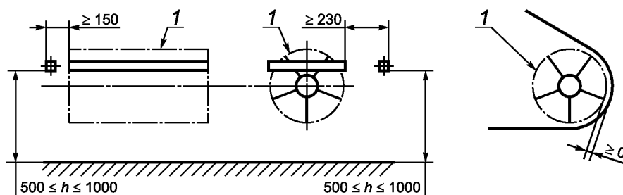
Рисунок 14 — Подбирающий механизм
