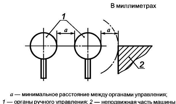
Рисунок 1 — Расстояние между органами управления
