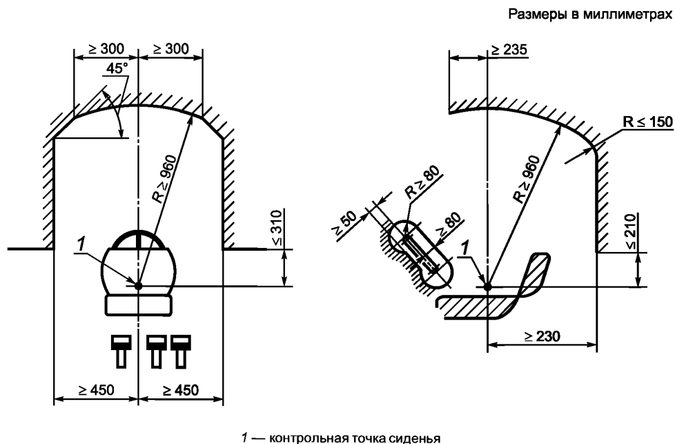
Рисунок 7 — Размеры внутреннего пространства кабины
