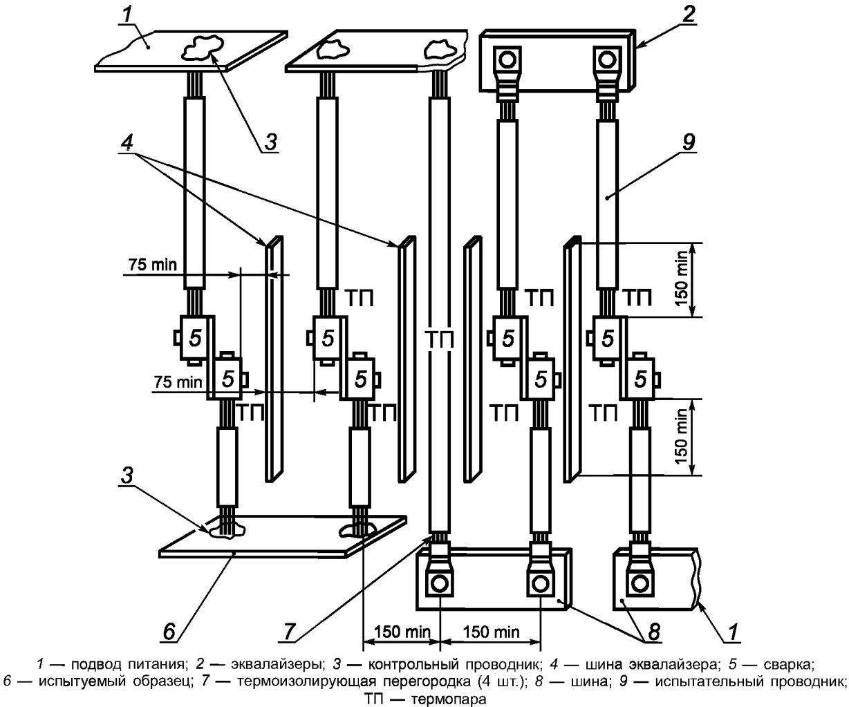
Рисунок L.1 — Испытательное устройство
