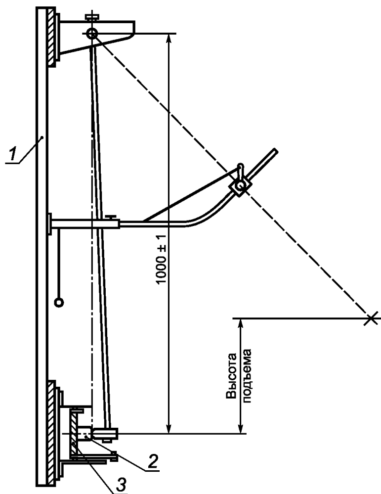
1 — опора; 2 — образец; 3 — монтажная опора
