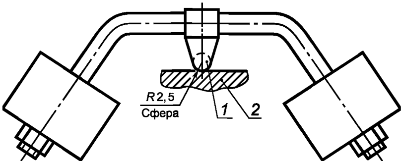
1 — стальной шарик; 2 — испытуемый образец
