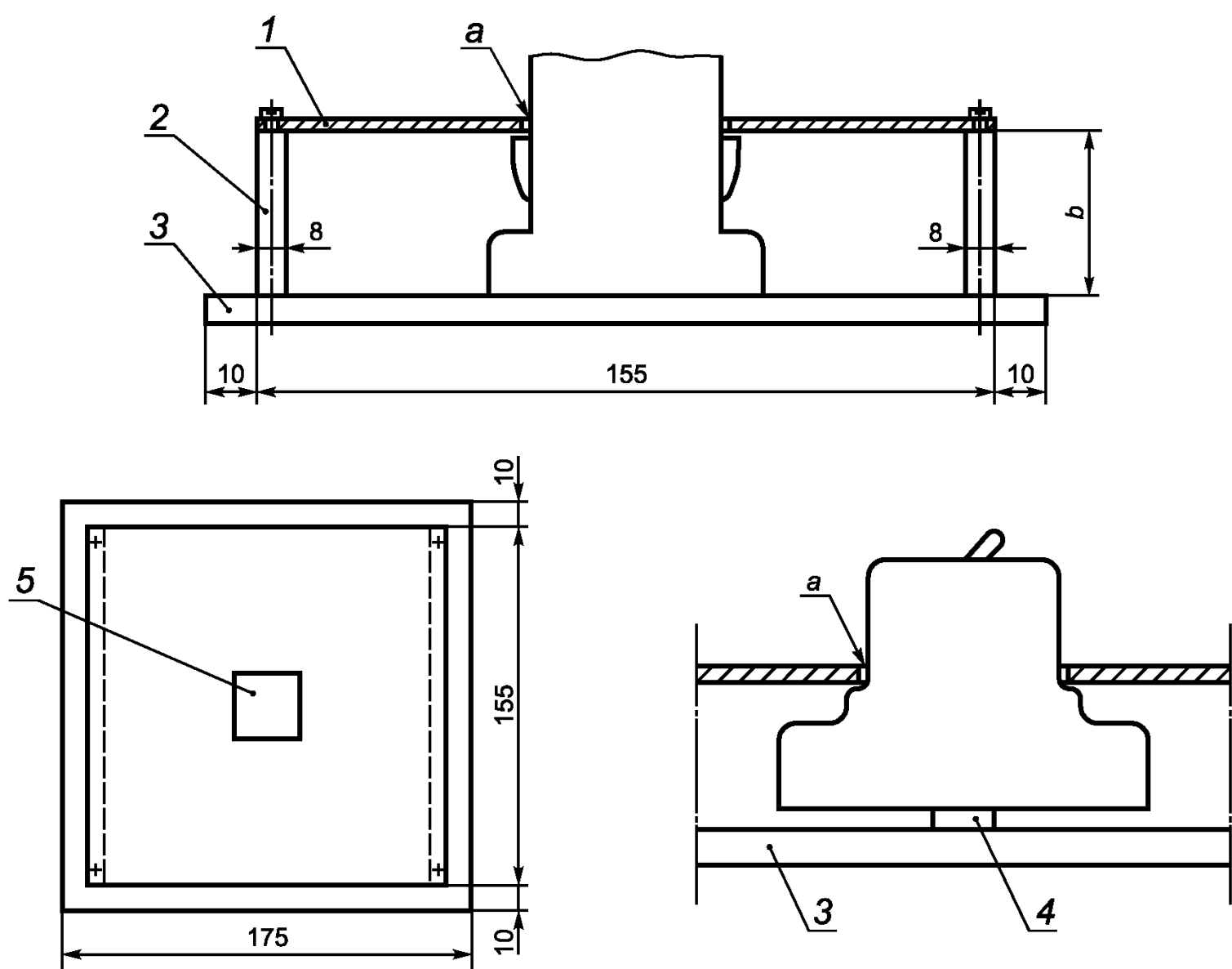
1 — съемная стальная панель толщиной 1 мм; 2 — алюминиевые листы толщиной 8 мм; 3 — монтажная плита; 4 — рейка для установки выключателей реечного монтажа; 5 — окно в панели для выхода выключателя: a — зазор между краями окна в панели и корпусом автоматического выключателя должен составлять 1—2 мм; b — высоту алюминиевых листов следует выбирать так, чтобы стальная панель опиралась на выступы корпуса выключателя, а при их отсутствии обеспечивался зазор 8 мм между панелью и частями выключателя, находящимися под напряжением и требующими защиты дополнительной крышкой, расположенной снаружи панели
