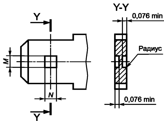
Допуск расположения углублений относительно центральных осей штекера 0,13 мм.
