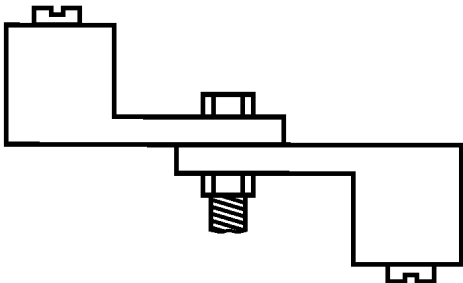
Рисунок L.1 — Испытательное устройство
