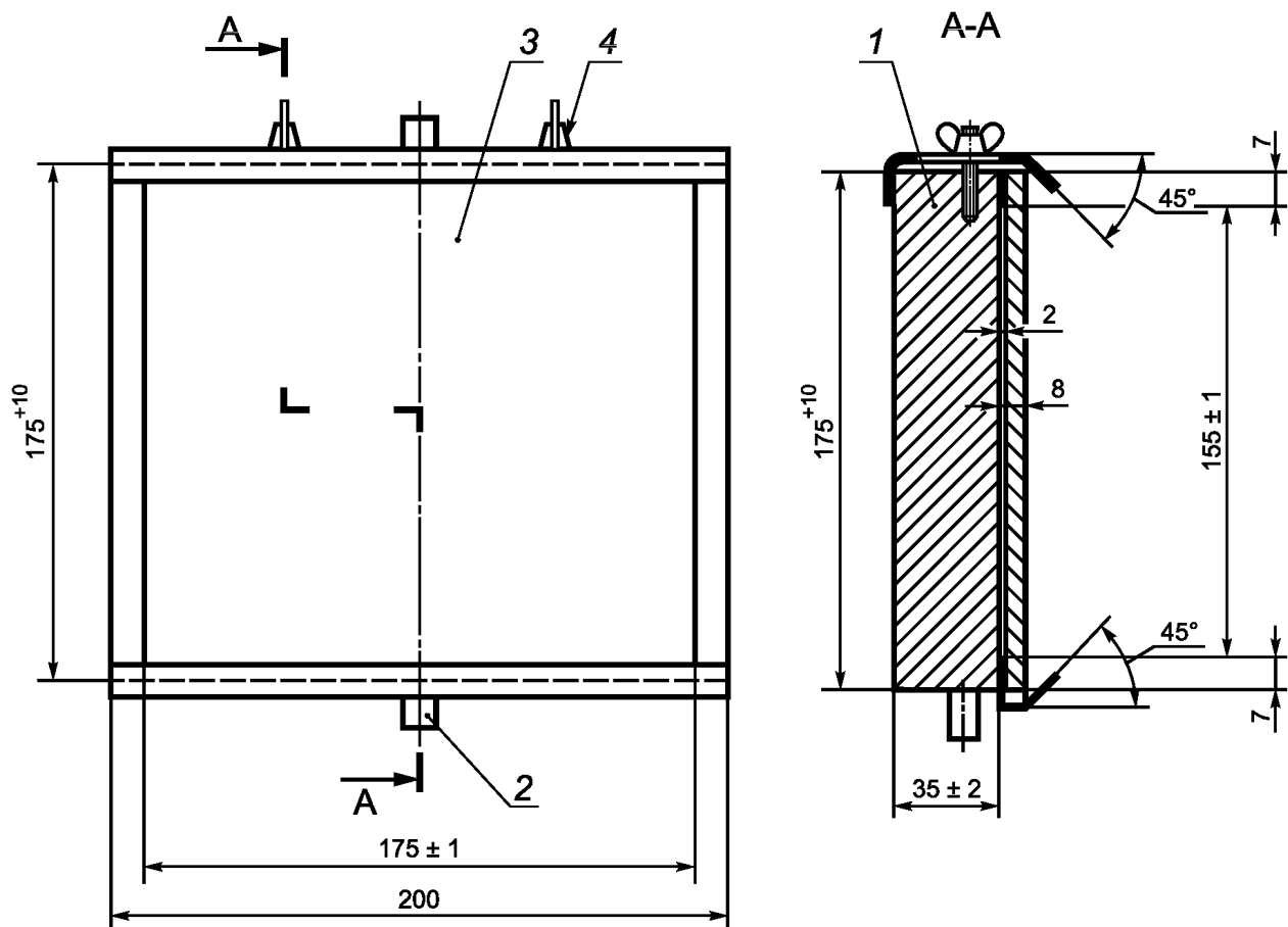
1 — главная опора массой (10 \pm 1) кг; 2 — стержень для поворота вокруг вертикальной оси; 3 — монтажная опора (из древесины — для настенной установки; для других типов монтажа см. рисунки 13 и 14); 4 — зажимы для поворота в горизонтальной плоскости
