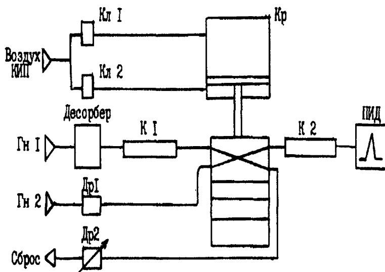
Рис. 2. Схема «вырезки».
