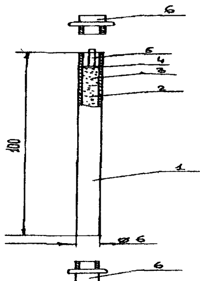
Рис. 1. Колонка накопительная.
