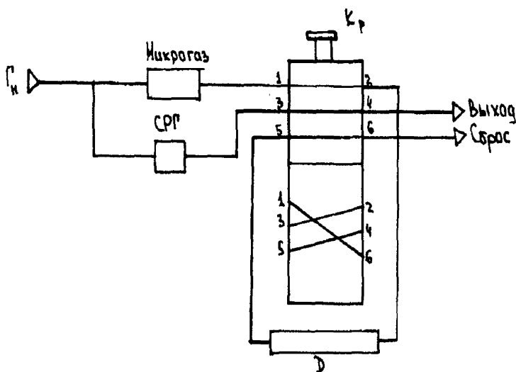
Рис. 4. Схема отбора градуировочной смеси.
