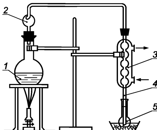
Рисунок 1 — Прибор для перегонки спирта
