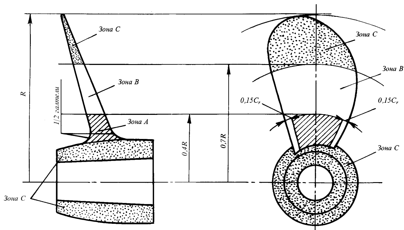
Рис. 9.1.3.2
