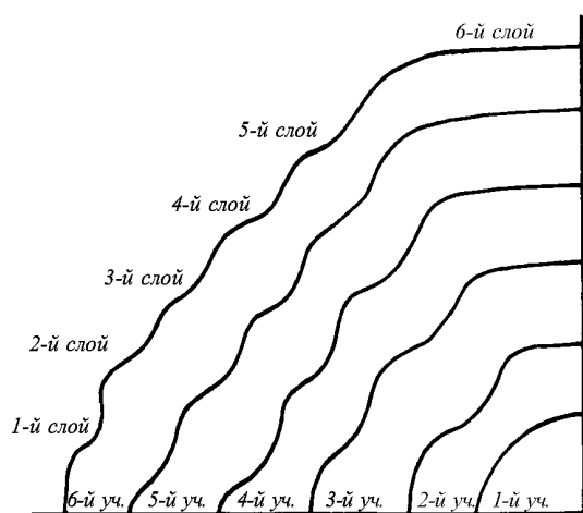
Рис. 9.1.7.34 Валики наплавки
