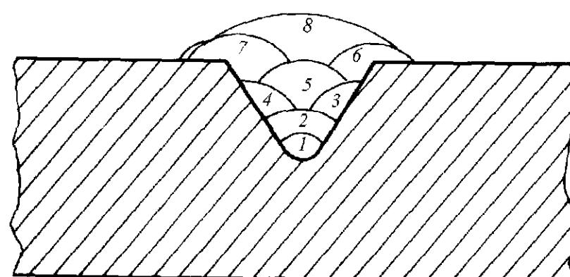
Рис. 9.2.10.16-1 Очередность наложения сварных швов при наплавке
