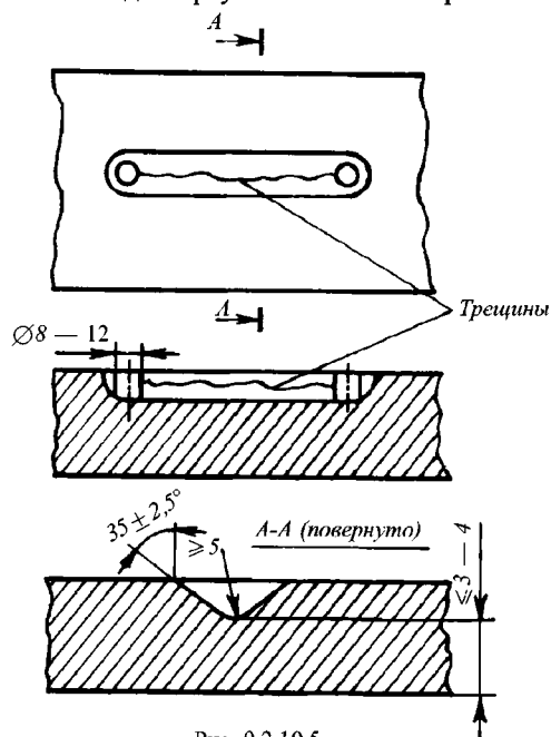
Рис. 9.2.10.5 Подготовка под заварку несквозных трещин
