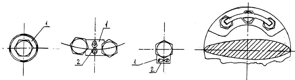
Рис. 9.1.13.8 Варианты стопорения гаек для шпилек съемных лопастей:
