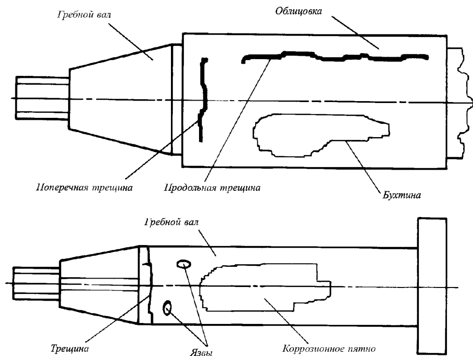
Рис. 8.6.1.1 Типовые повреждения гребных валов
