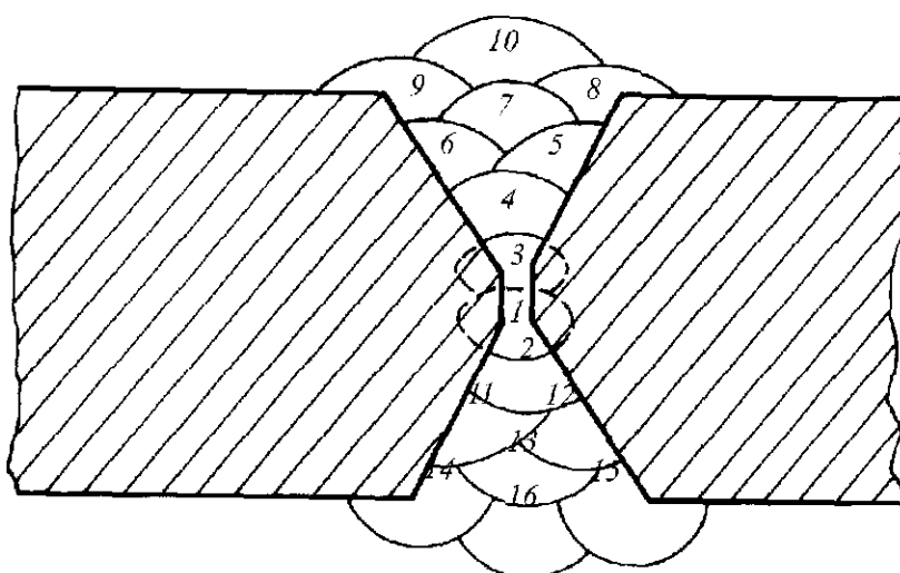
Рис. 9.2.10.16-2 Очередность наложения сварных швов в зависимости от вида разделки
