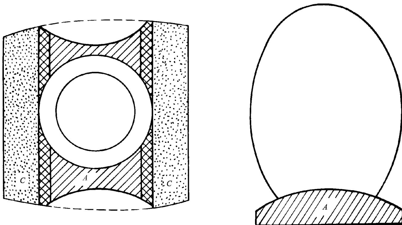
Рис. 9.2.3.2-2
