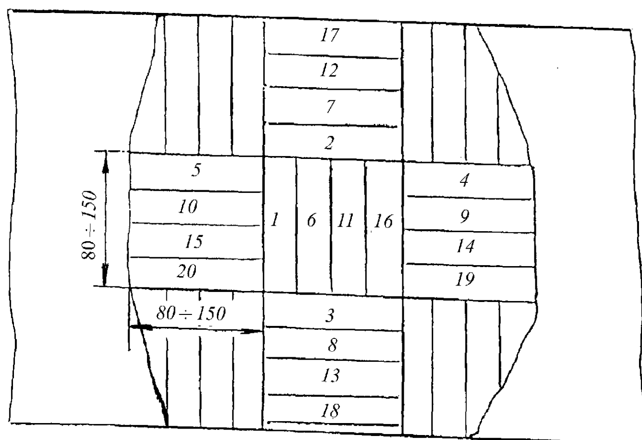
Рис. 9.2.10.16-1 Очередность наложения сварных швов при наплавке
