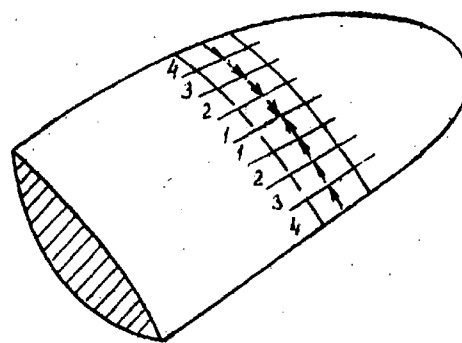
Рис. 9.1.7.20-2 Приварка наделок
