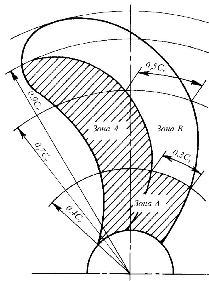
Рис. 9.1.3.5
