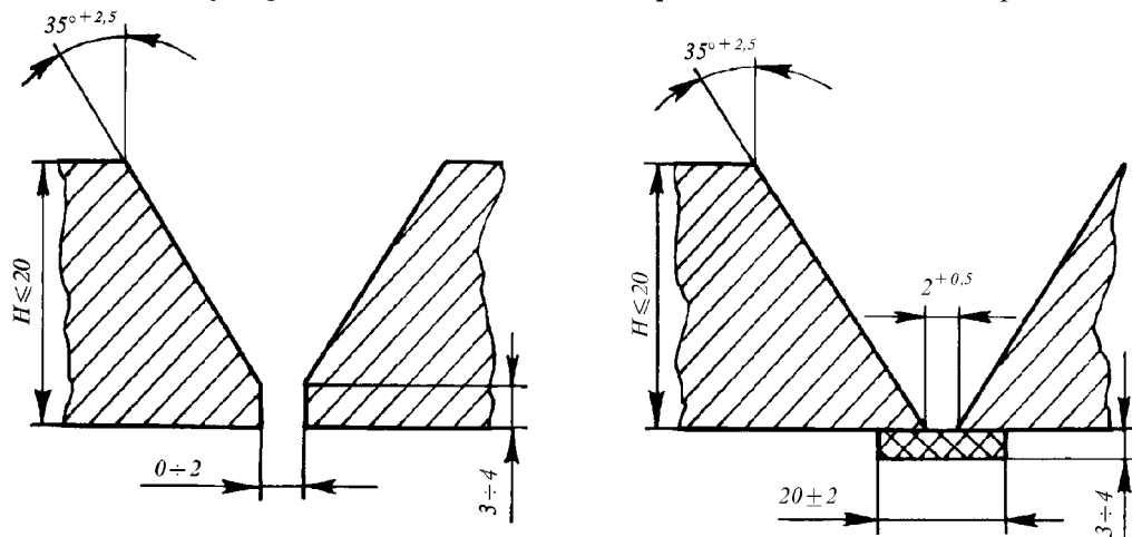
Рис. 9.2.10.8-1 V-образная разделка кромок
