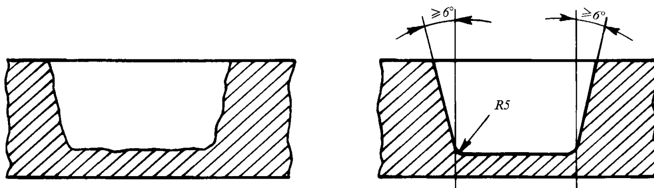
Рис. 9.1.7.16-3 Углы разделки широких раковин
