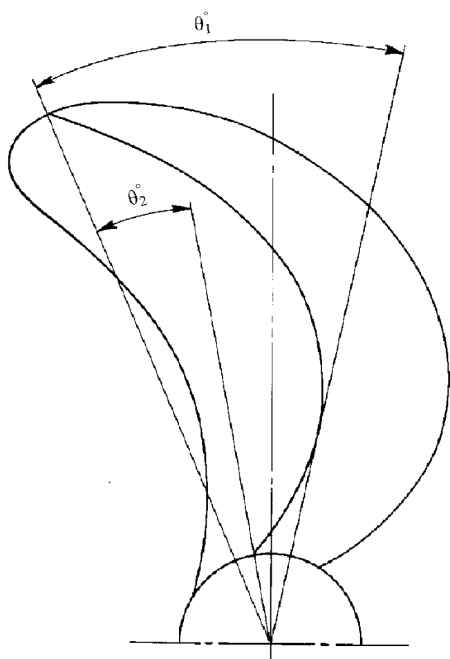
Рис. 9.1.3.4:
