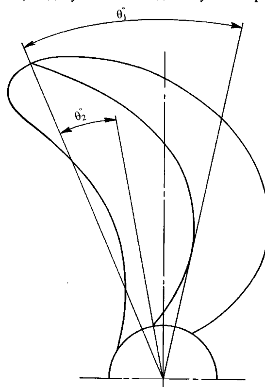
Рис. 9.2.3.3-2
