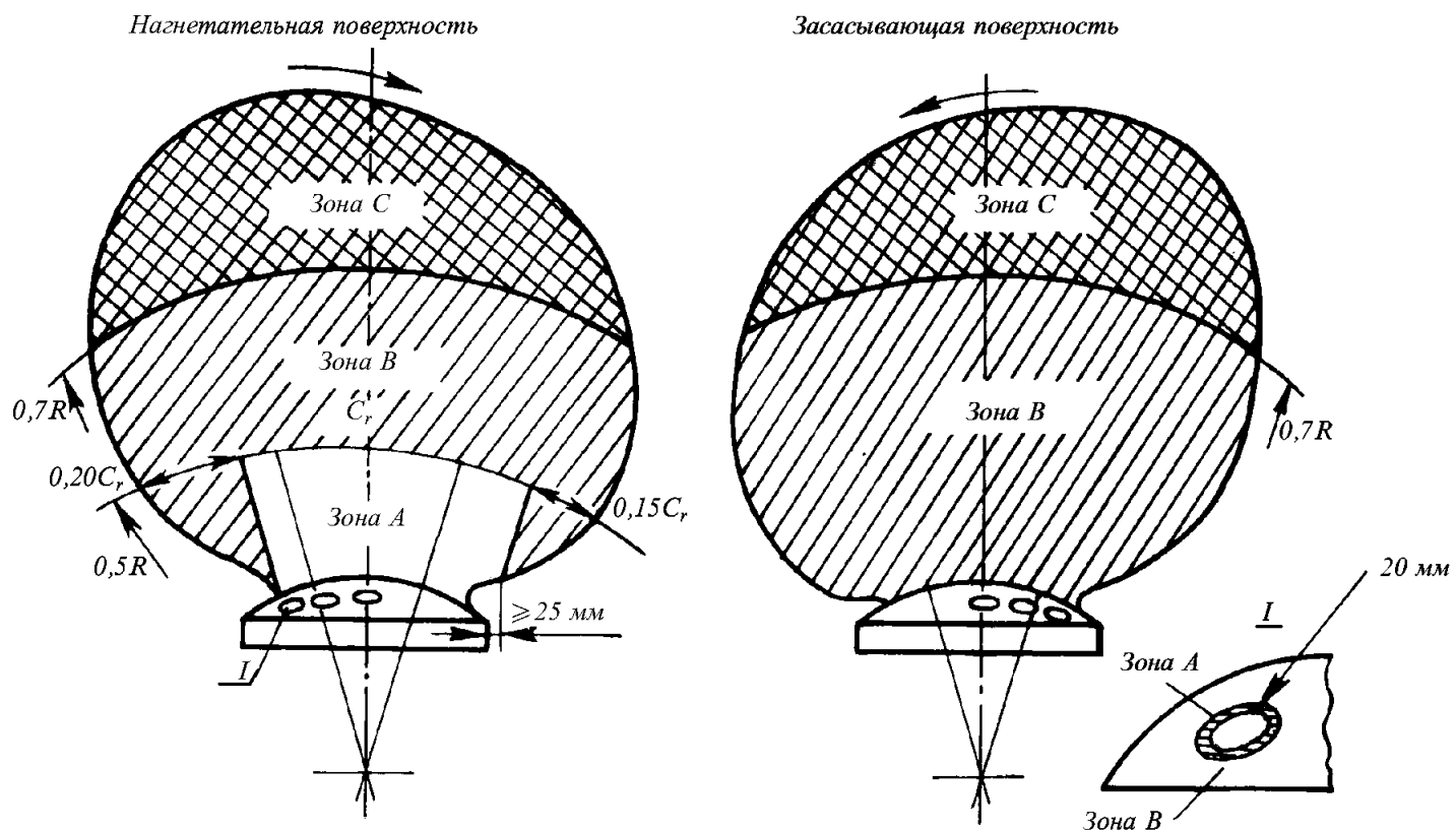
Рис. 9.2.3.2-1
