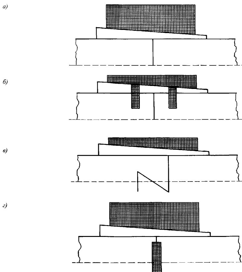
Рис. 8.8.3.1
