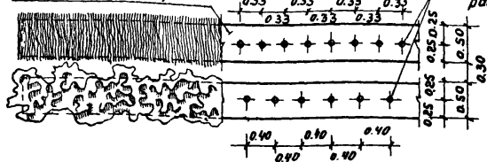
Траншея для изгороди
