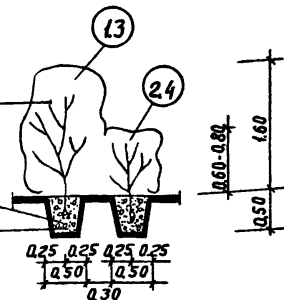
Траншея для двухрядной живой изгороди
