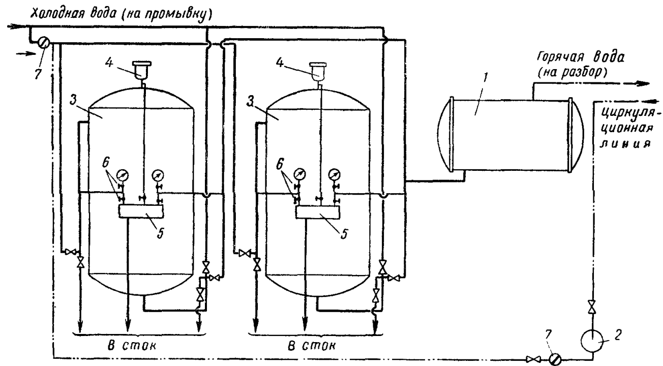
Рис. 3. Принципиальная схема подключения магмассовых фильтров к трубопроводам холодной воды (до водонагревателя)
