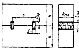
Рис 5. Схема соединения на пластинчатых нагелях
