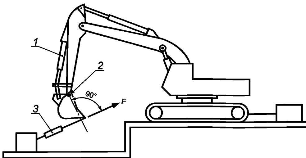
а) Гидравлический экскаватор с ковшом «обратная лопата»
