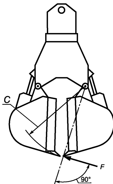
Рисунок 7 — Рабочий орган захват (рейфер). Расчет усилия замыкания (см. 5.2.4)
