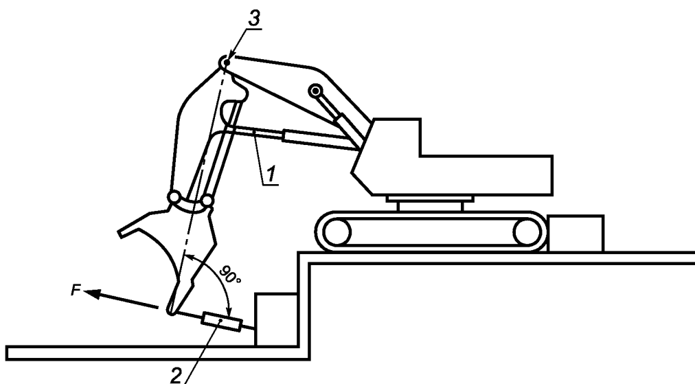
б) Гидравлический экскаватор с ковшом «прямая лопата»
