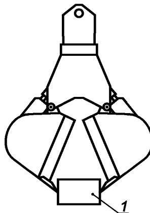
1 — динамометр
