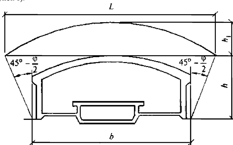
Рисунок 1 - Схема для расчета высоты свода обрушения
