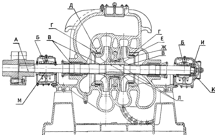
Рисунок 14 - Насос ЦН 3000 - 197
