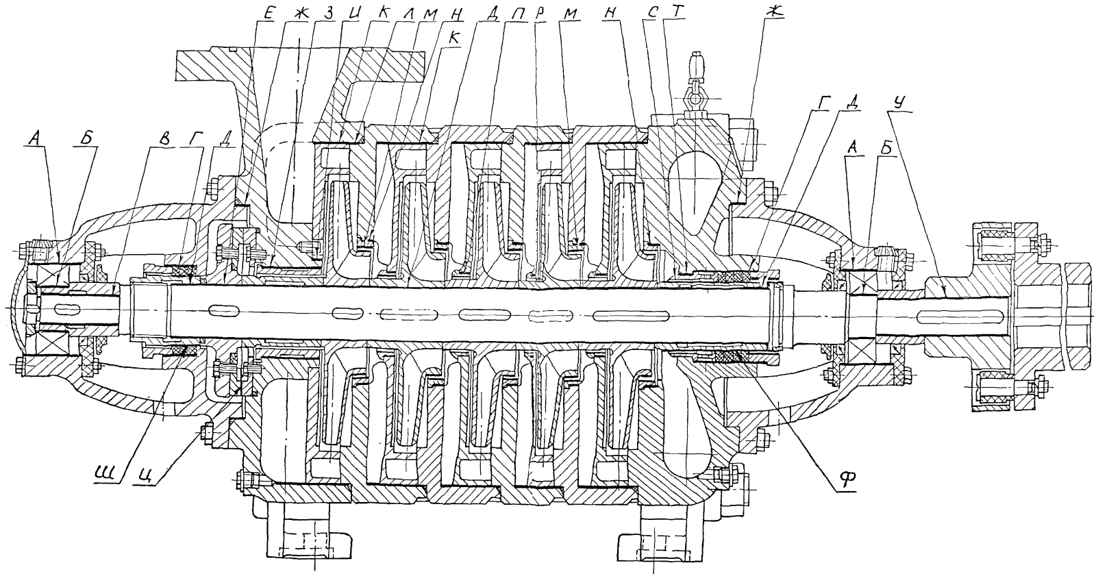
Рисунок 4 - Насосы ЦНС 180-85...425
