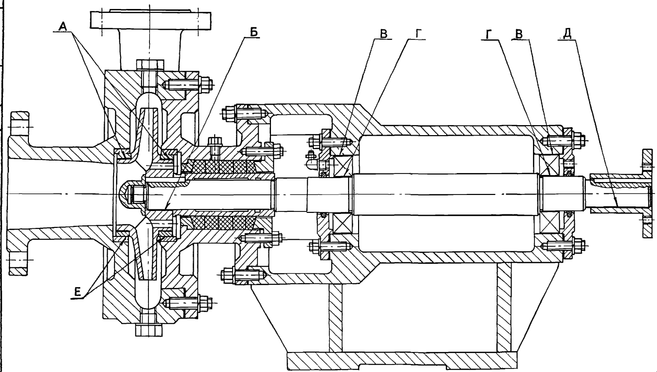
Рисунок 12 - Насос К 45/55
