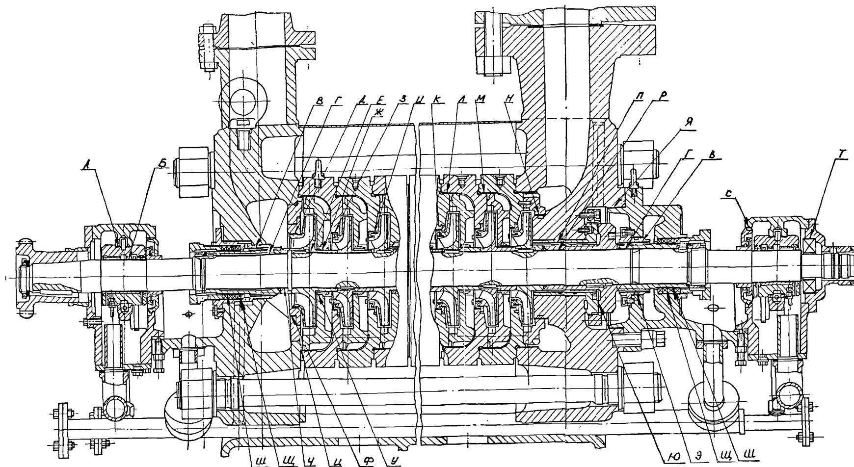
Рисунок 5 - Насос ЦНС 180-1422
