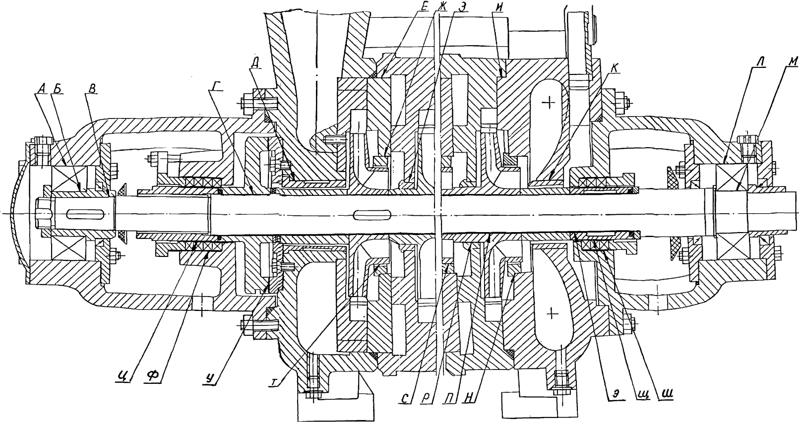
Рисунок 3 - Насосы ЦНС 105-98...490
