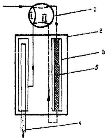
Рис. 2: Схема устройства для ввода пробы в хроматограф.
