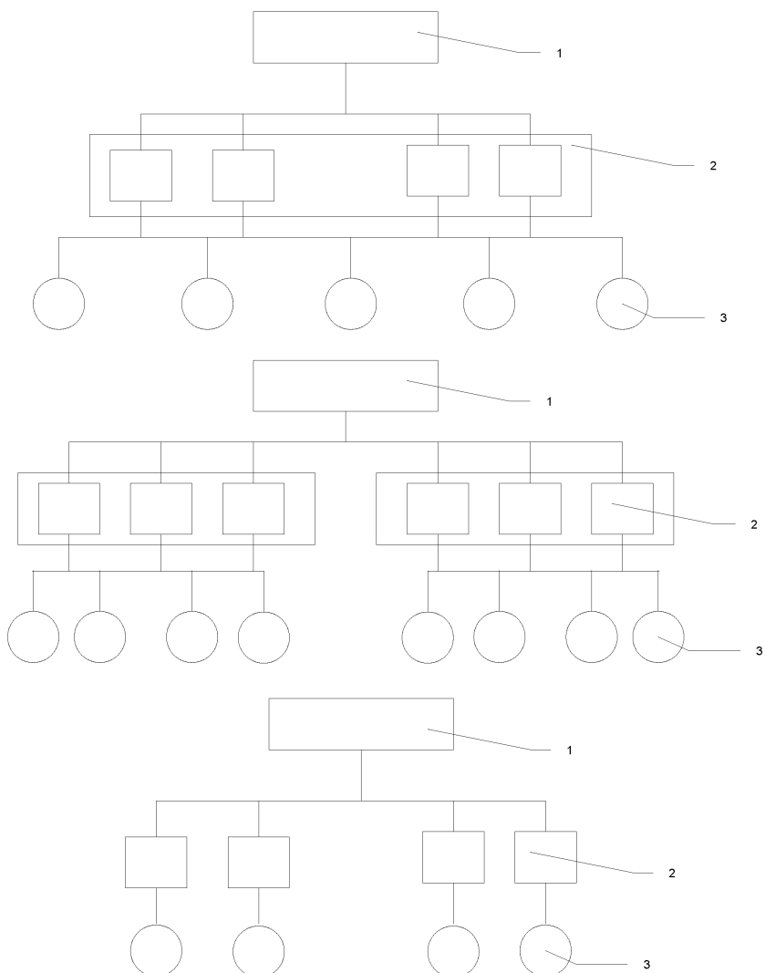
Рисунок В.5. Компоновка воздушной системы отжата: объединенные (общестанционные)- верхняя схема, групповые (блочные)- средняя схема и индивидуальные (агрегатные)- нижняя схема.
