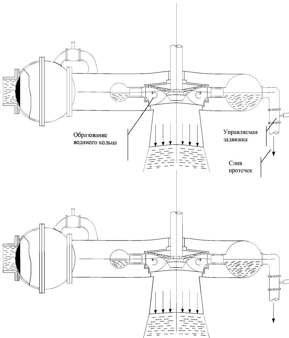
Рисунок В.3. Схема отжата воды для гидроагрегата, оснащенного рабочим колесом с коэффициентом быстроходности менее 150
