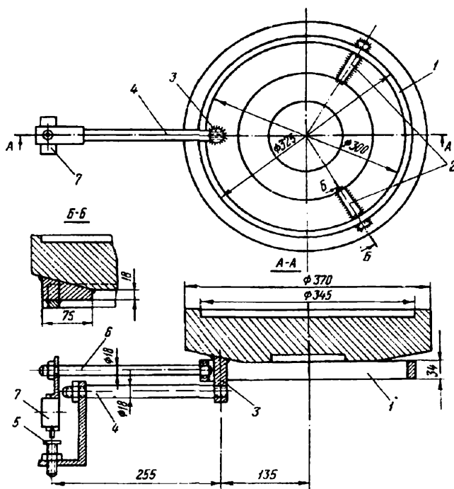
1 - кольцо; 2 - ребра-приварыши; 3 - стержень; 4 - нижний рычаг с уголком; 5 - винт с опорной поверхностью; 6 - верхний рычаг; 7 - индикатор
