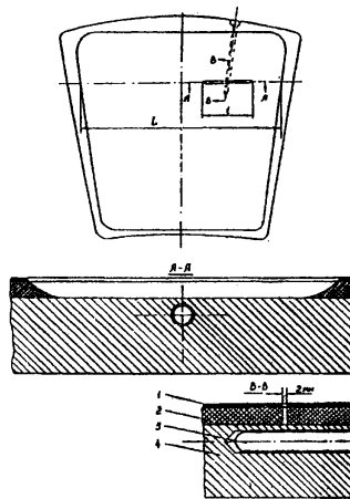
Рисунок Д.6 – Выполнение пазов на ЭМП-сегментах для повышения чувствительности термоконтроля.
