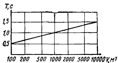
Рис. 4. Зависимость оптимального времени реверберации от объема учебного помещения
