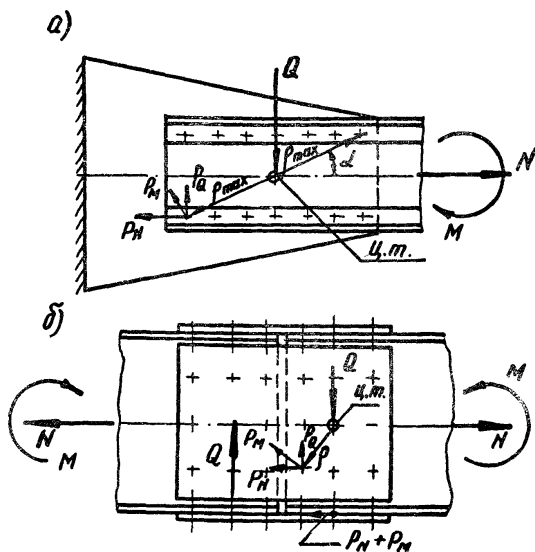
а - узловое прикреплeние; б - стык.
