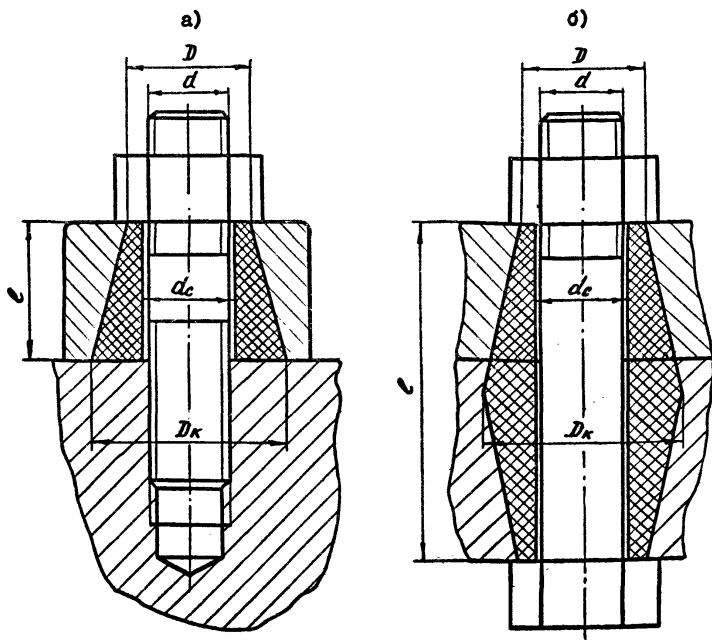
а- шпилька; б- болт
