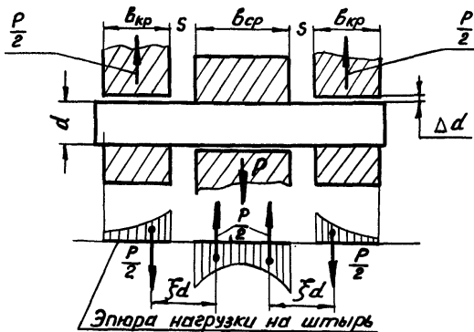
Fd - расстояние между равнодействующими Черт. 5.3
