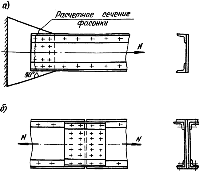
а - узловое приращение; б - стык.
