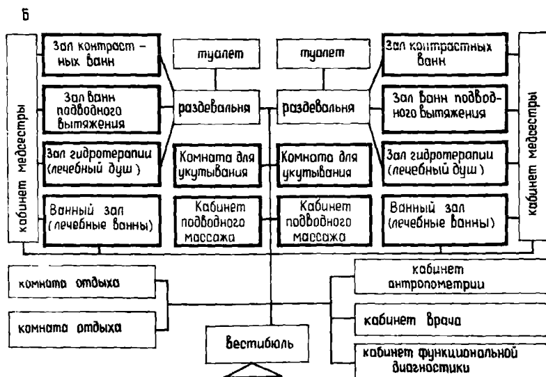
Рис. 5. Рекомендуемые схемы взаимосвязи помещений гидротерапевтической группы а – при ВЛОК типа I, II; б – при ВЛОК типа II, III
