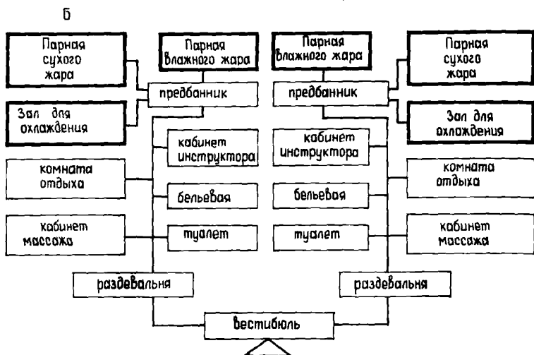
Рис. 7. Рекомендуемые схемы взаимосвязи группы помещений сауны а — при ВЛОК типа I; б — при ВЛОК типа II, III
