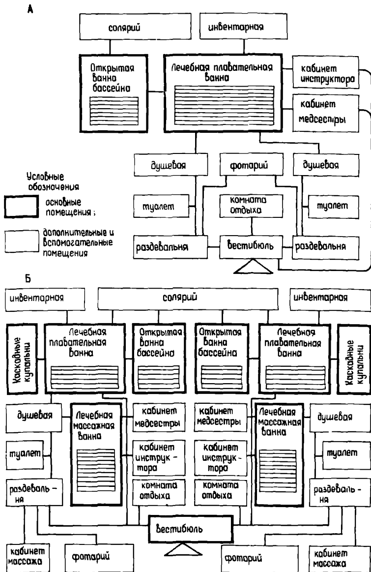
Рис. 3. Рекомендуемые схемы взаимосвязи группы помещений лечебно-го бассейна а – при ВЛОК типа I, II; б – при ВЛОК типа II, III
