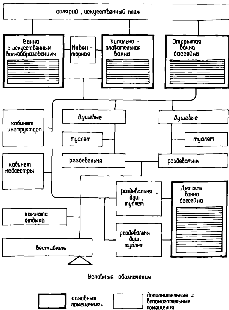
Рис. 4. Рекомендуемая схема взаимосвязи групп помещений купально-оздоровительного бассейна при ВЛОК типа Ц, Ш
