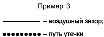
Рисунок А.1а — Путь утечки и воздушный зазор для пазов с параллельными стенками и пазов V-образной формы
