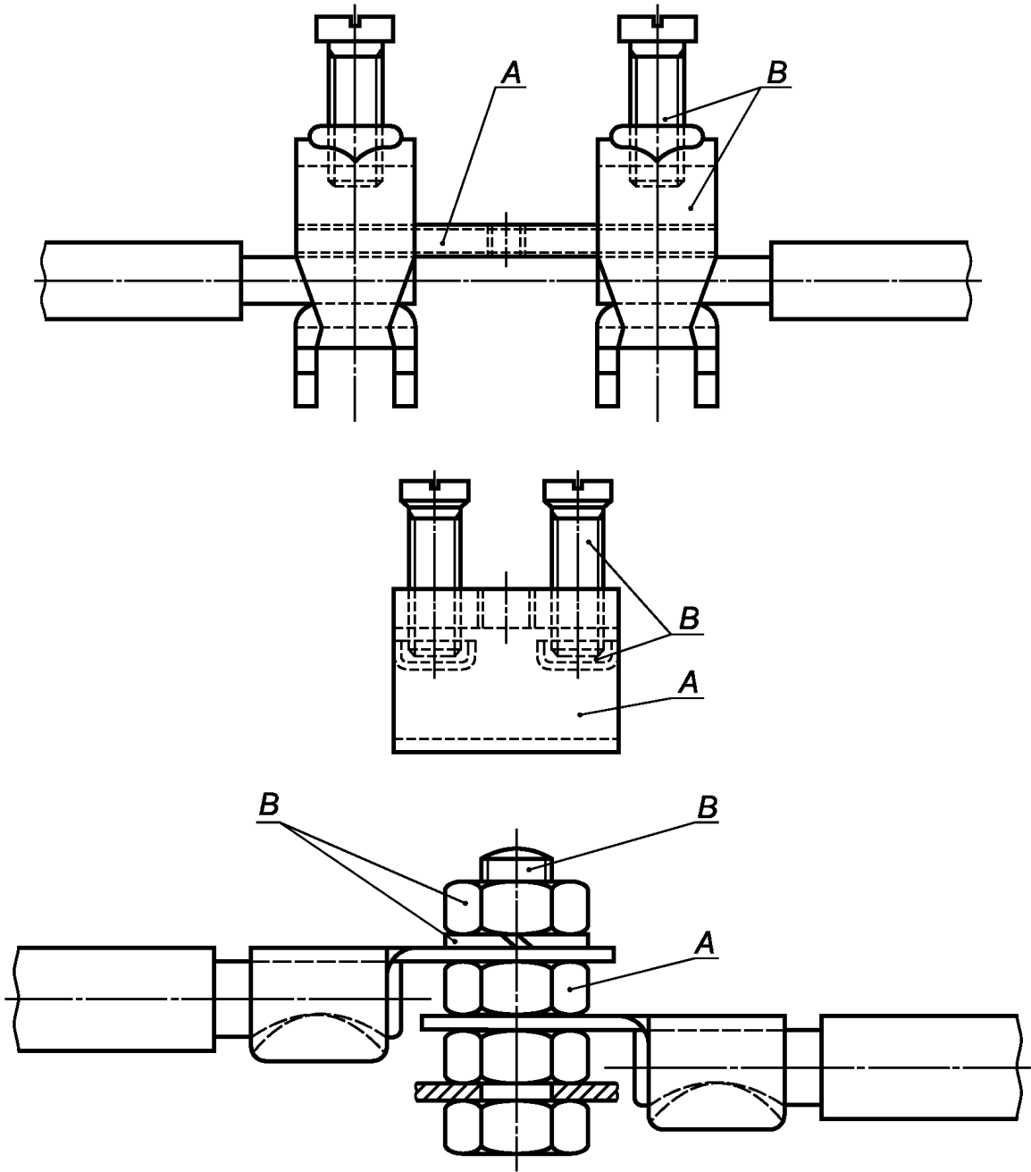
A — токопроводящая часть, обеспечивающая непрерывность заземления; B — часть, обеспечивающая или передающая контактное давление
