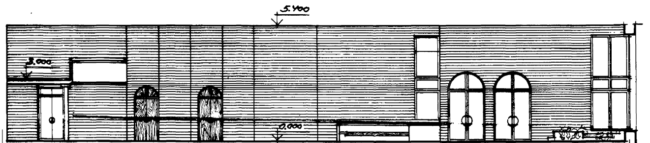
развёртка стены в осях "14-Е"
