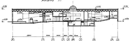
разрез 1-1
