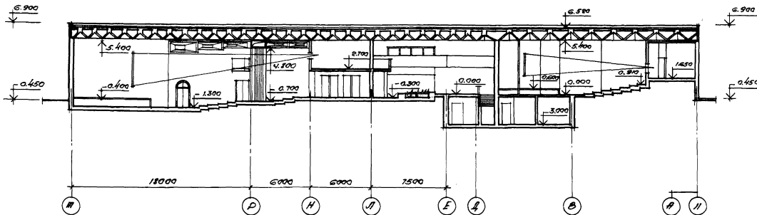
разрез 2-2
