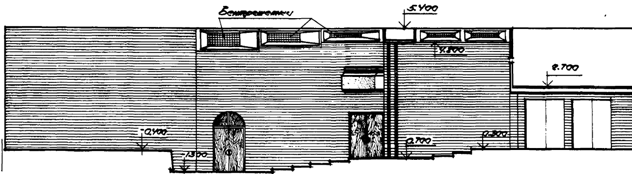
развёртка стены в осях "17-Д"
