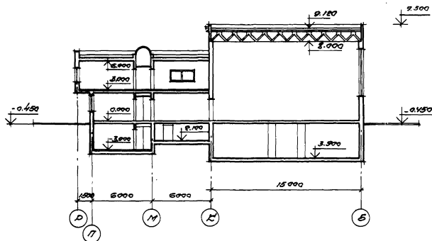
разрез 3-3
