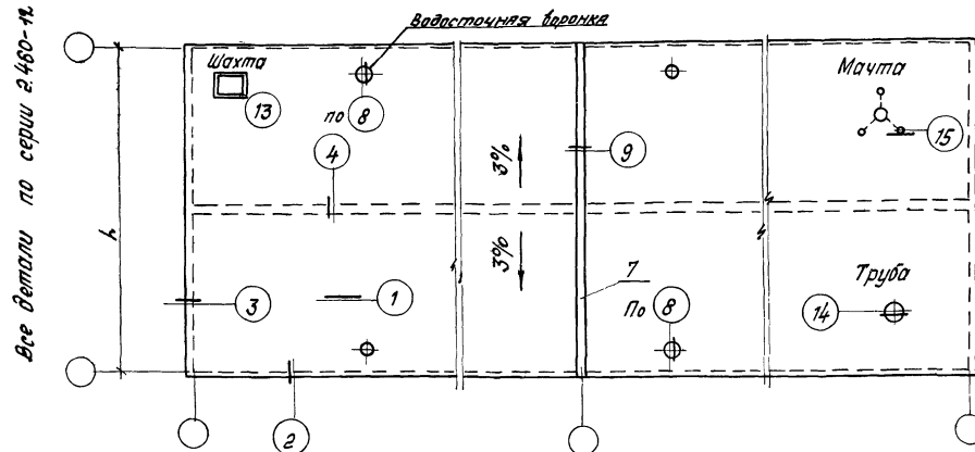
Схема маркировки конструкций и деталей кровли
