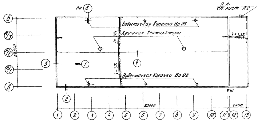
План кровли
