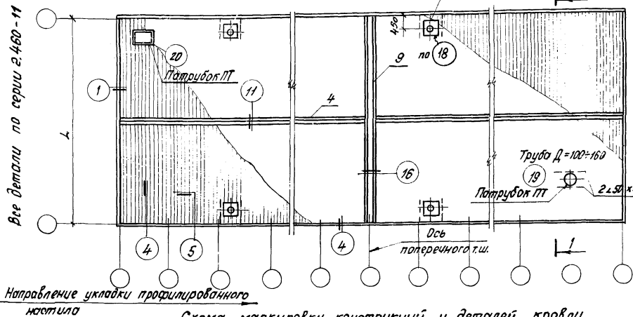
Схема маркировки конструкций и деталей кровли
