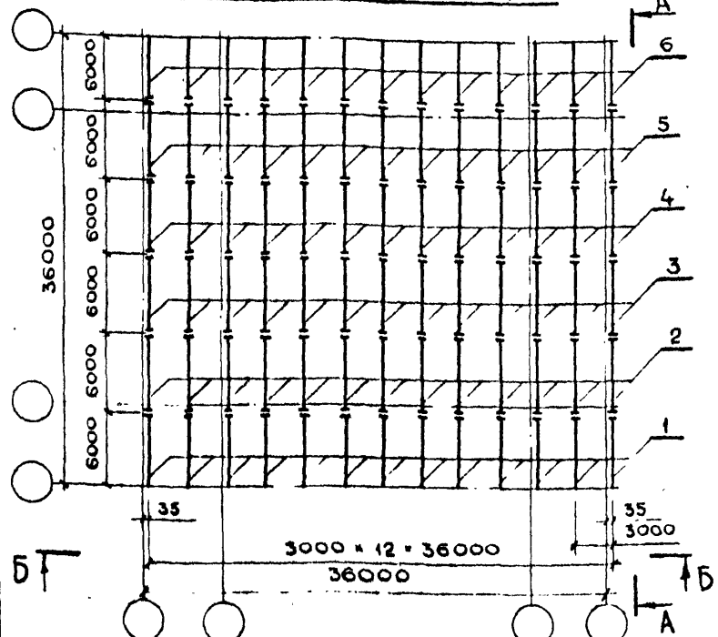
МОНТАЖНАЯ СХЕМА ПРОГОНОВ ЗДАНИЯ ИЗ ДВУХ И БОЛЕЕ СЕКЦИЙ
