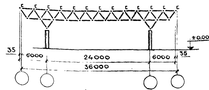
МОНТАЖНАЯ СХЕМА ПРОГОНОВ ЗДАНИЯ ИЗ ДВУХ И БОЛЕЕ СЕКЦИЙ
