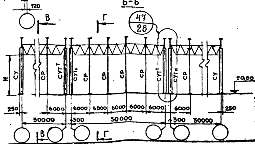
МОНТАЖНАЯ СХЕМА СТОЕК ФАХВЕРКА ЗДАНИЙ С СЕКЦИЯМИ 30x30 м. Ключ подбора стоек фахверка
