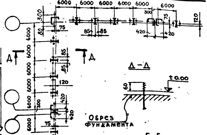
ПЛАН АНКЕРНЫХ БОЛТОВ СТОЕК ФАХВЕРКА
