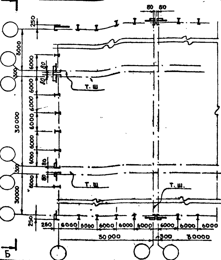
МОНТАЖНАЯ СХЕМА СТОЕК ФАХВЕРКА ЗДАНИЯ ИЗ ДВУХ И БОЛЕЕ СЕКЦИЙ
