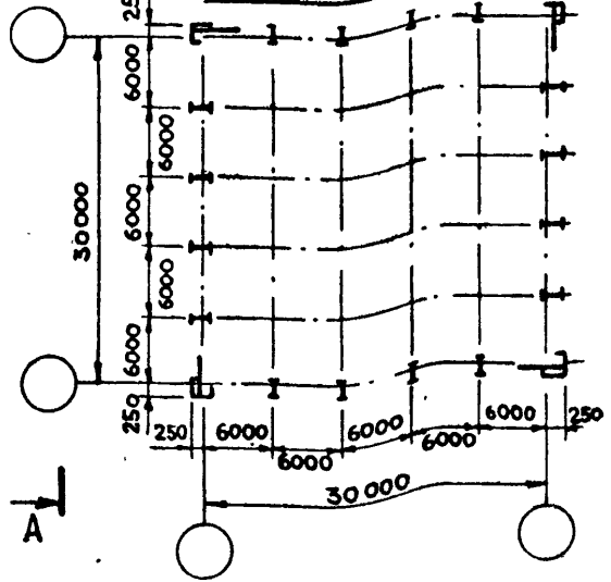
МОНТАЖНАЯ СХЕМА СТОЕК ФАХВЕРКА ЗДАНИЯ ИЗ ДВУХ И БОЛЕЕ СЕКЦИЙ
