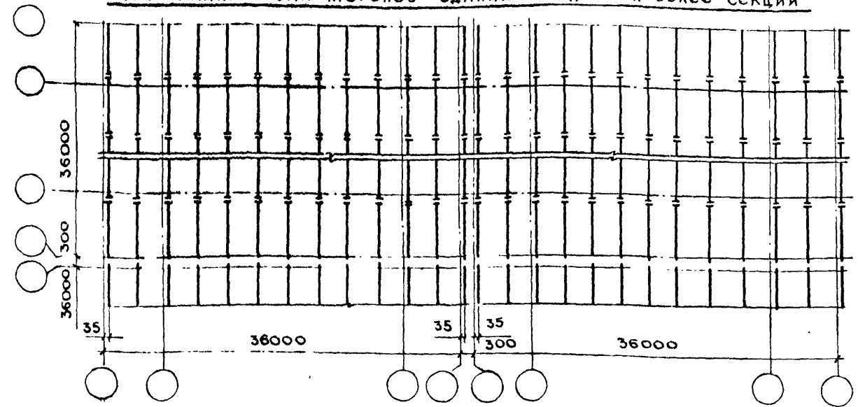
МОНТАЖНАЯ СХЕМА ПРОГОНОВ ЗДАНИЯ ИЗ ДВУХ И БОЛЕЕ СЕКЦИЙ
