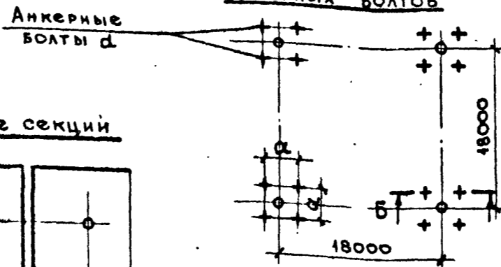
ПЛАН КОЛОН И АНКЕРНЫХ БОЛТОВ
