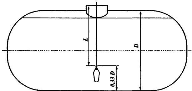
Рис. 1. Схема отбора проб нефтепродуктов из железнодорожных цистерн
