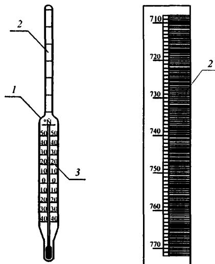
Рис. 3. Ареометр:
