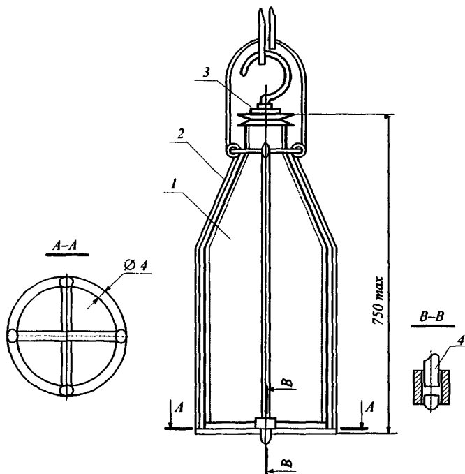
Рис. 2. Переносной пробоотборник:
