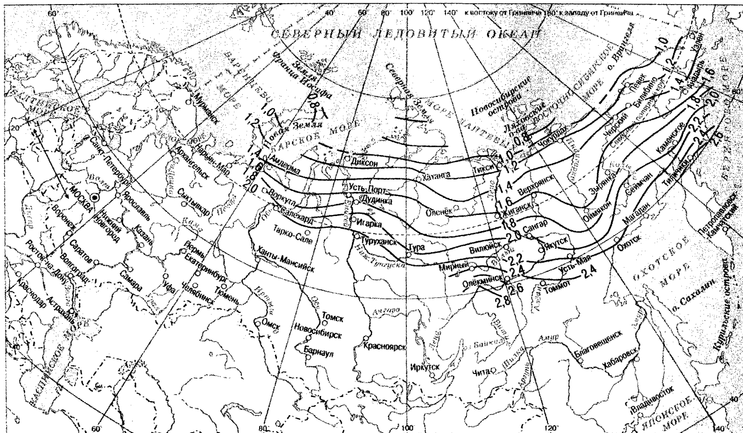
Рисунок Г.2 – Глубины оттаивания глинистых грунтов
