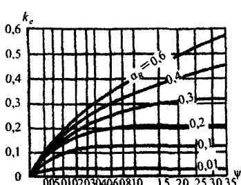
Рисунок К.2 – Графики для определения коэффициентов \xi_e и k_e
