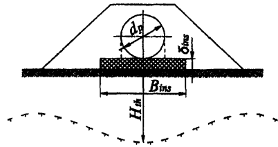
Рисунок Н.1 – Расчетная схема для определения глубины многолетнего оттаивания ММГ под теплыми и горячими трубопроводами, проложенными подземно (а) и наземно (б)
