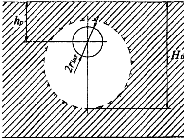
Рисунок Н.1 – Расчетная схема для определения глубины многолетнего оттаивания ММГ под теплыми и горячими трубопроводами, проложенными подземно (а) и наземно (б)
