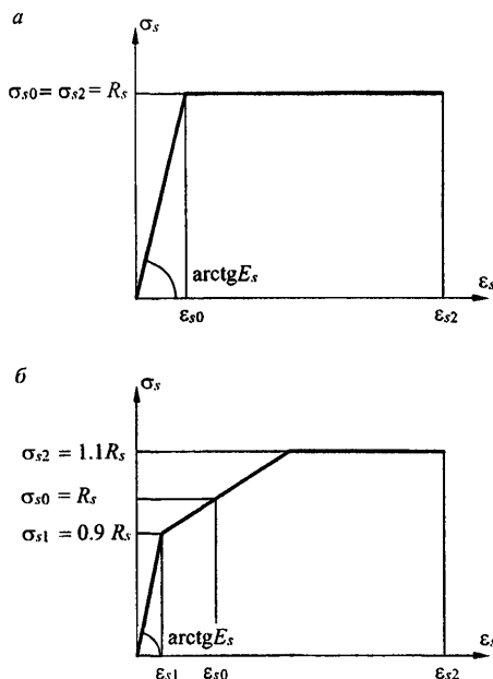
a – двухлинейная диаграмма; б – трехлинейная диаграмма
