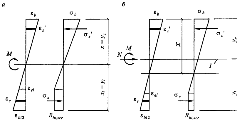
I – Уровень центра тяжести приведенного поперечного сечения
