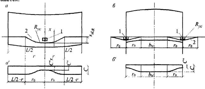
a – расположение источника замачивания под серединой (прогиб) здания; a' – схема изменения коэффициента жесткости при прогибе здания; b – расположение источников замачивания по торцам (выгиб) здания; b' – схема изменения коэффициента жесткости при выгибе здания; 1 – источники замачивания грунтов; 2 – кривые просадок грунта от собственного веса
