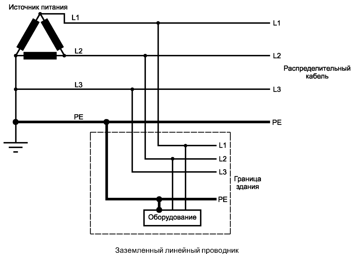
Рисунок J.1 — Примеры системы энергоснабжения TN-S
