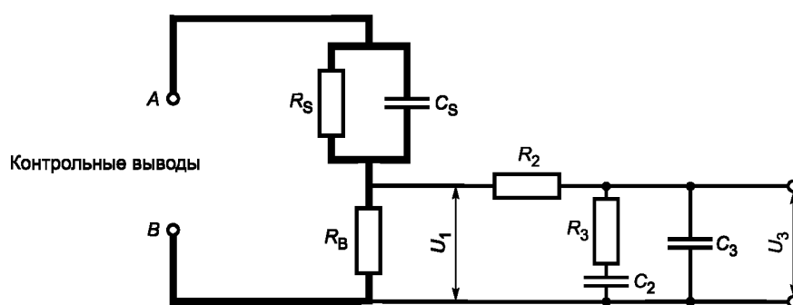
Рисунок 4 — Измерительная схема. Ток прикосновения, взвешенный для ощущения и физиологической реакции
