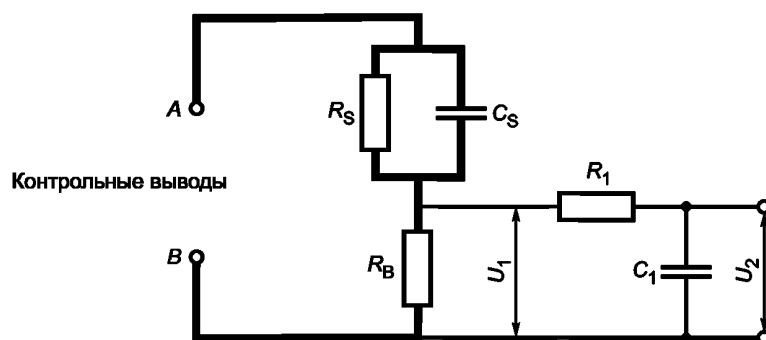
Рисунок 3 — Измерительная схема. Невзвешенный ток прикосновения
