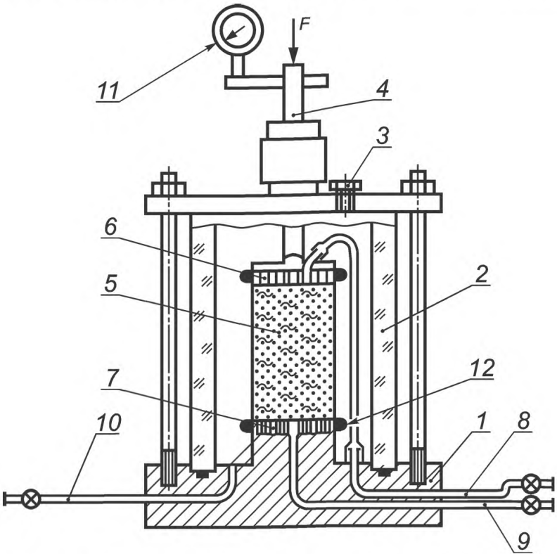
1 — основание камеры; 2 — корпус камеры; 3 — вентиль для выпуска воздуха; 4 — шток; 5 — образец грунта в оболочке; 6 — верхний штамп; 7 — нижний штамп; 8, 9 — магистрали системы дренажа, противодействия и измерения порового давления; 10 — магистраль давления в камере; 11 — индикатор перемещений; 12 — уплотняющее кольцо; F — нагрузка
