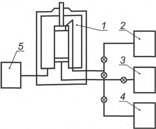
1 — камера прибора трехосного сжатия; 2 — блок измерения порового давления; 3 — блок противодействия; 4 — блок дренажа; 5 — блок давления в камере
