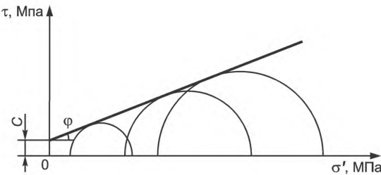
Диаграмма Кулона—Мора
